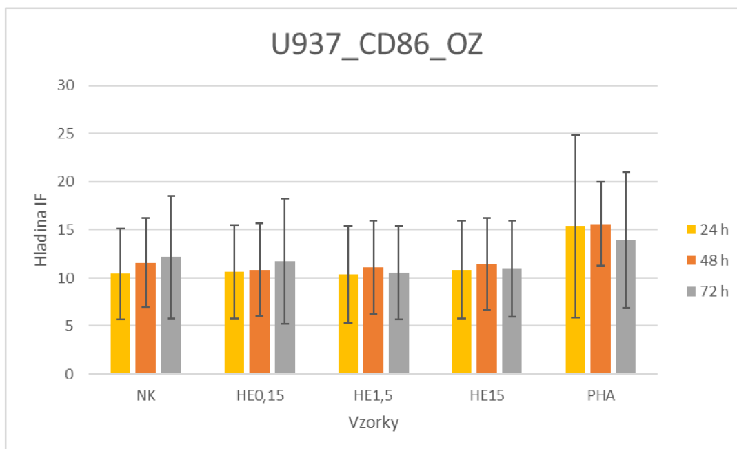
Graf 8: Hodnota imunofluorescence u buněčné linie U937 při použití markeru CD86 a ozáření gama zářením 2 Gy. Údaje představují průměrnou hodnotu \pm směrodatná odchylka. Zkratky: NK = negativní kontrola, HE0,15 = vzorek s hovězím extraktem o koncentraci 0,15 mg/ml, HE1,5 vzorek s hovězím extraktem o koncentraci 1,5 mg/ml, HE15 = vzorek s hovězím extraktem o koncentraci 15 mg/ml, PHA = phytohaemagglutinin, IF = imunofluorescence, OZ = ozářené vzorky.
