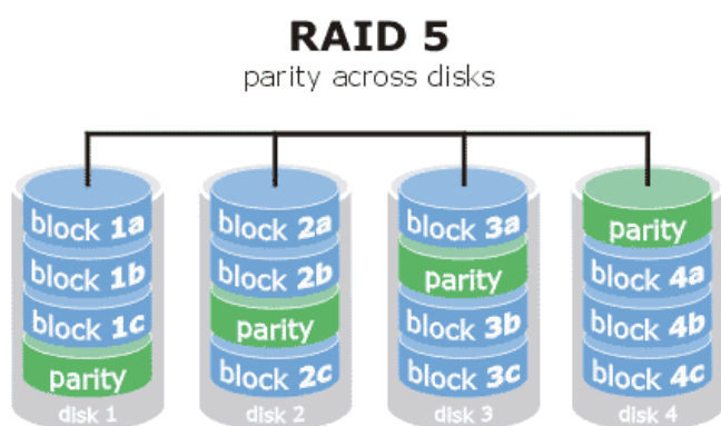
Obrázek č. 4 Schéma uložení dat RAID 5 [Zdroj: http://www.hdd-tool.com/raid/raid-5-features-advantage-and-disadvantage.htm ]
