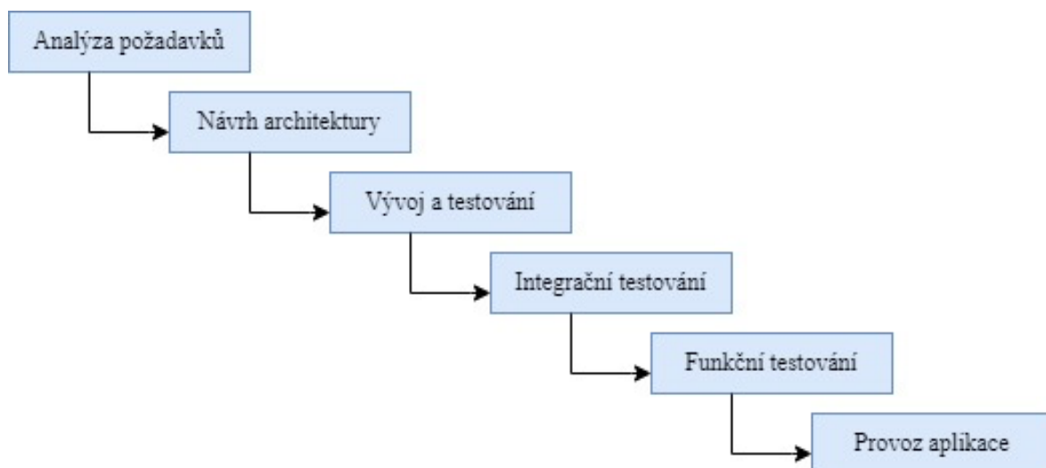
Obrázek 6 Vodopádový model
