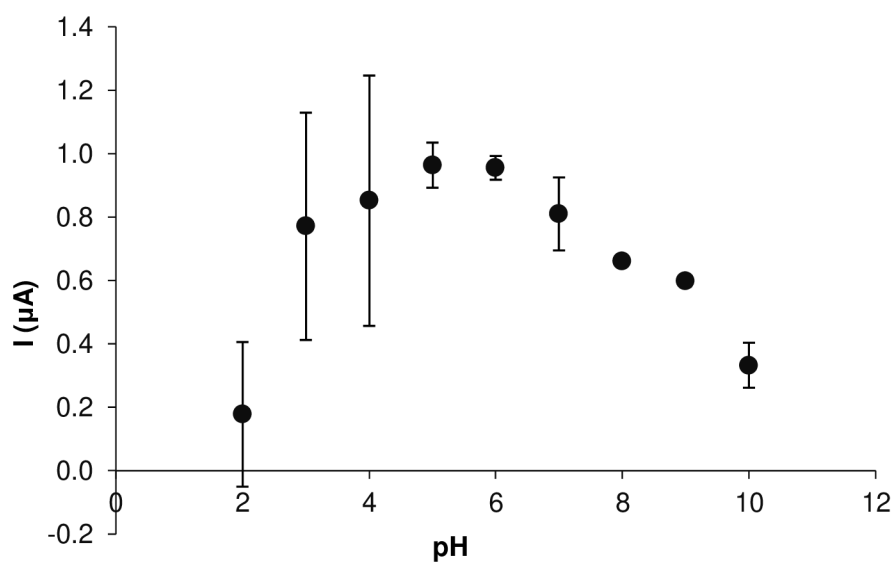
Obr. 13 - Závislost odezvy kodeinu na pH elektrolytu
