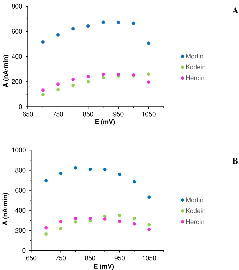
Obr. 16 - Hydrodynamické voltamogramy morfinu, kodeinu a heroínu získané EC detekcí na kanálu ECD1 (A) a kanálu ECD2 (B)
