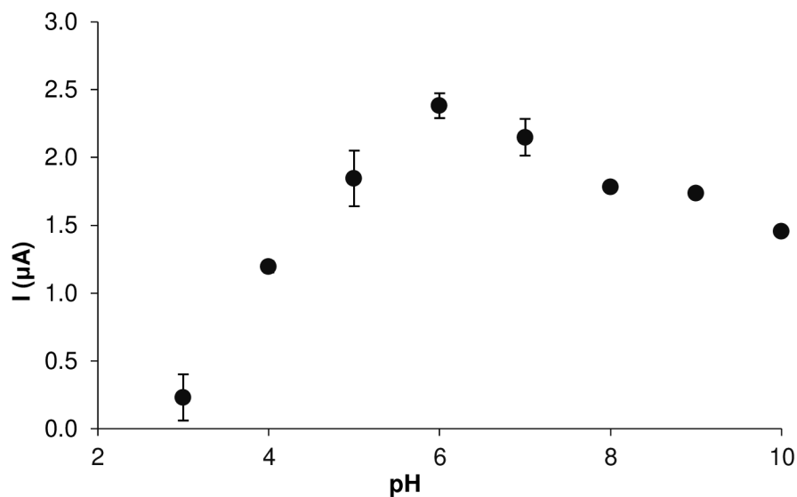
Obr. 12 - Závislost odezvy heroinu na pH elektrolytu
