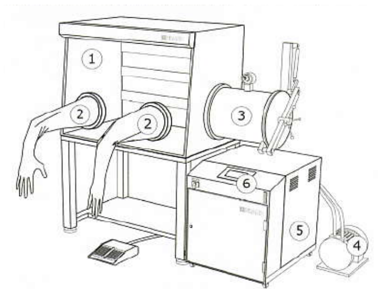
Obr.18: Drybox.
