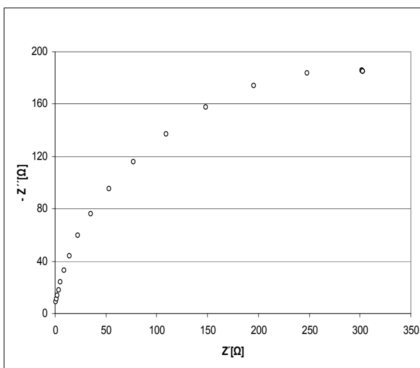
Obr. 35: Impedanční charakteristika pro LiClO 4 , Dimethylsulfoxid
