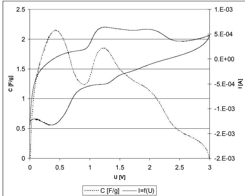
Obr. 26: Scan cyklické voltametrie I=f(U) pro \text{LiBF}_4 , Dimethylsulfoxid
