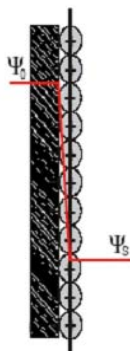
Obr. 1: Helmholtzův model elektrické dvojvrstvy ( \Psi_0 – velikost potenciálu na povrchu pevné fáze, \Psi_s – velikost potenciálu ve středu iontu na povrchu pevné fáze).
