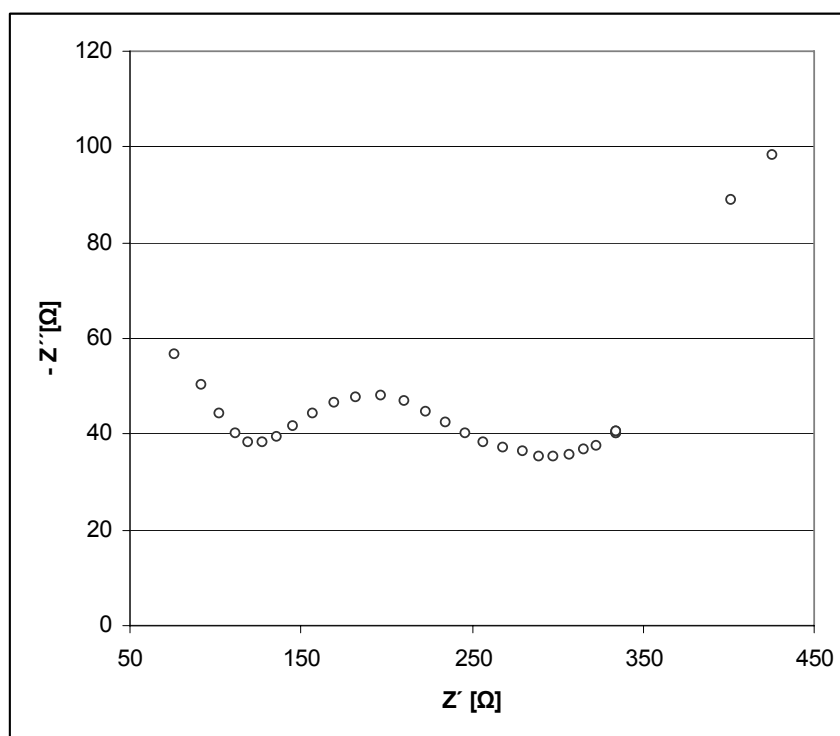
Obr. 34: Impedanční charakteristika pro LiClO 4 , Propylencarbonat
