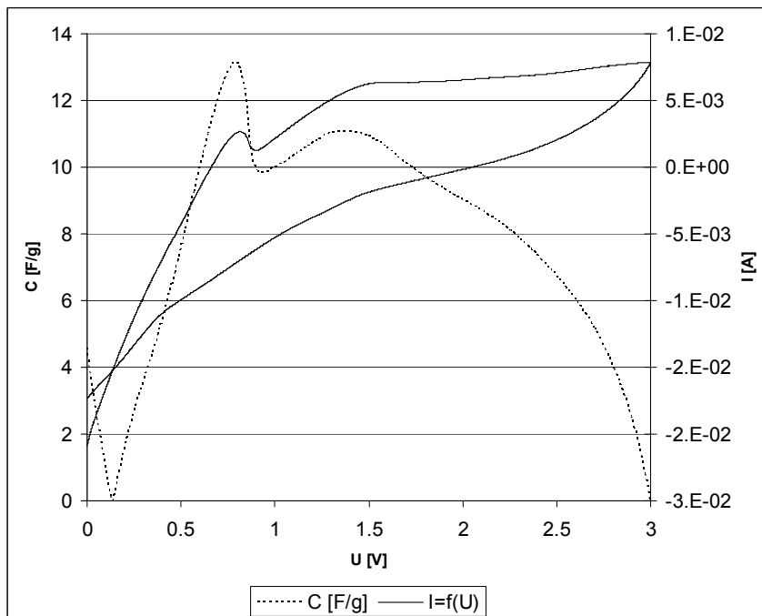
Obr. 29: Scan cyklické voltametrie I=f(U) pro LiPF 6 , Propylencarbonat
