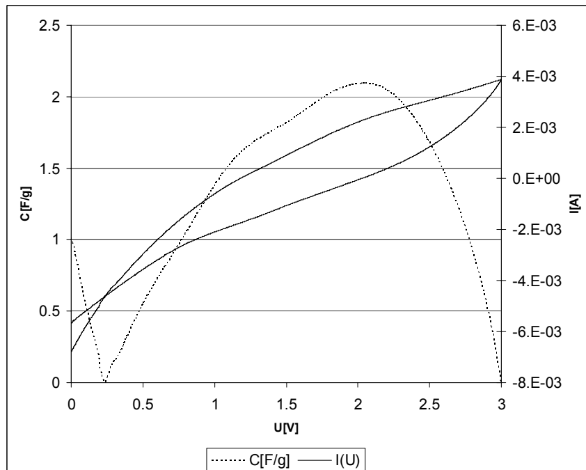
Obr. 27: Scan cyklické voltametrie I=f(U) pro \text{LiBF}_4 , Propylencarbonat
