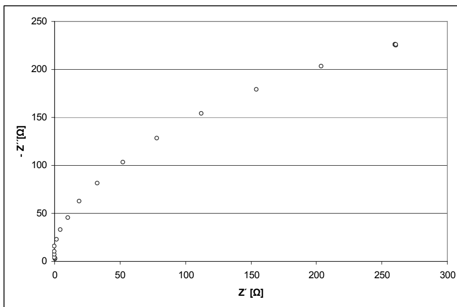
Obr. 38: Impedanční charakteristika pro LiBF 4 , Dimethylsulfoxid
