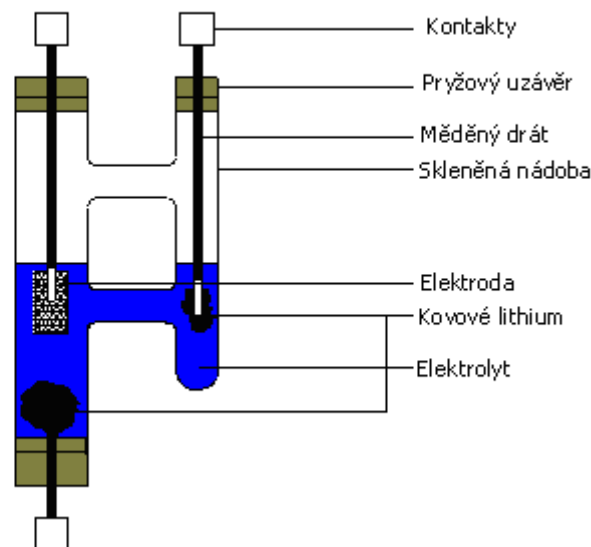
Obr.19: Spojitá nádobka
