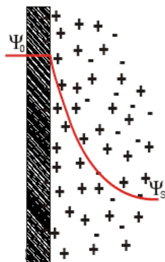
Obr.2: Gouyův-Chapmanův model elektrické dvojvrstvy ( \Psi_0 – velikost potenciálu na povrchu pevné fáze, \Psi_0 – velikost potenciálu ve vzdálenosti od povrchu pevné fáze).
