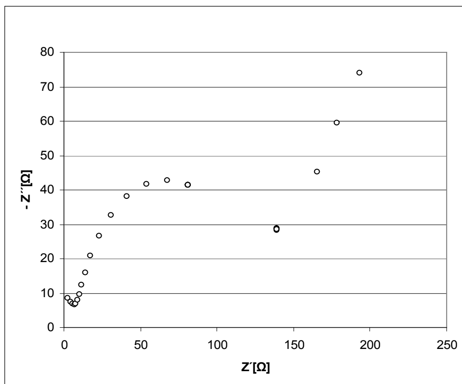
Obr. 38: Impedanční charakteristika pro LiBF 4 , Dimethylsulfoxid
