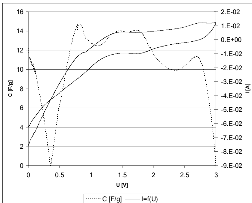
Obr. 30: Scan cyklické voltametrie I=f(U) pro LiPF 6 , Dimethylsulfoxid
