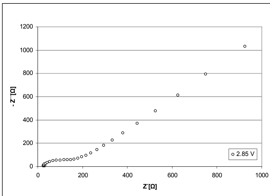
Obr. 36: Impedanční charakteristika pro LiBF 4 , Dimethylformamid
