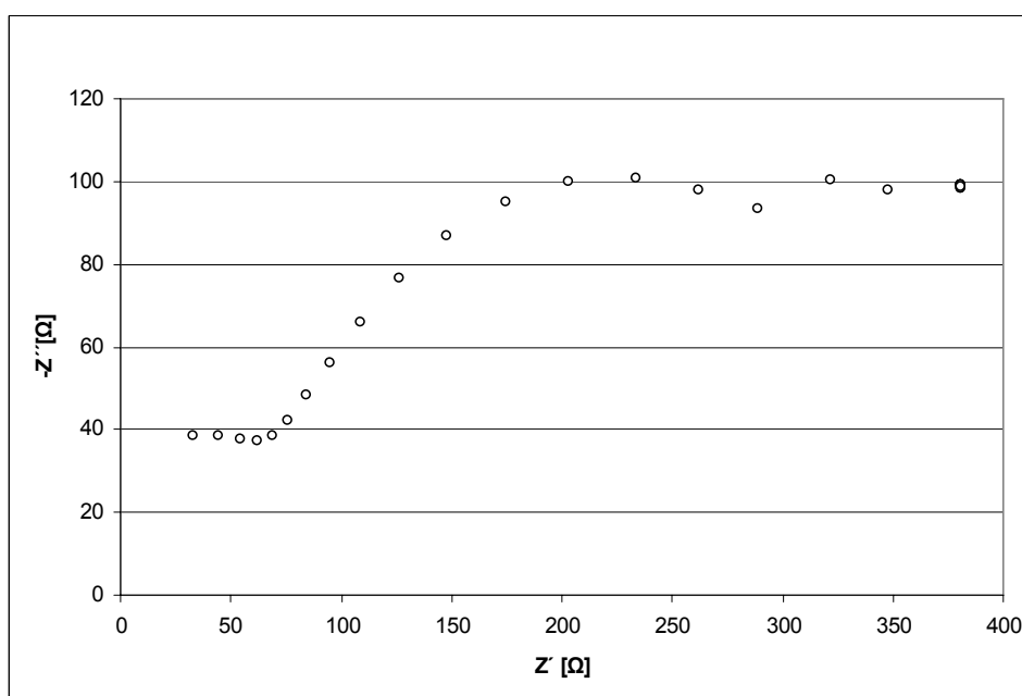
Obr. 37: Impedanční charakteristika pro LiBF 4 , Propylencarbonat
