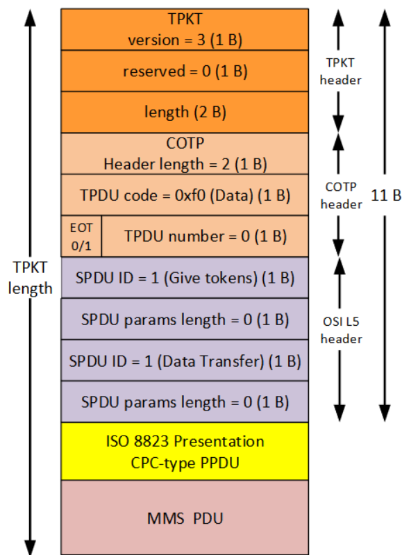
Obr. 5-5: Složení hlavičky [1]
