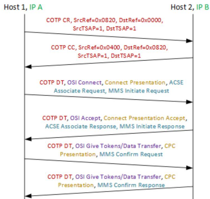
Obr. 4-2: Navázání spojení [1]
