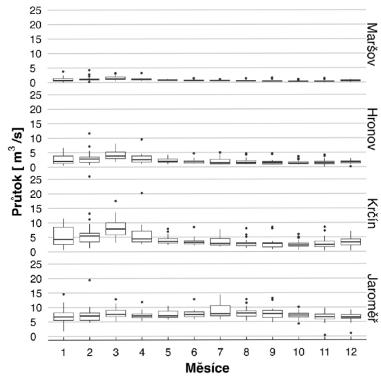
Obrázek 37: Krabicový graf modelovaného průtoku modelem TUW v měsíčních průměrných průtocích.
