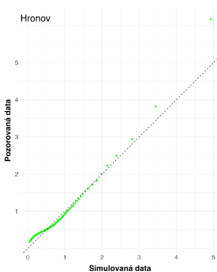
Obrázek 17: Rankitový graf zobrazující srovnání kvantilů měřených a simulovaných dat modelem BILAN na povodí měrné stanice v Hronově.
