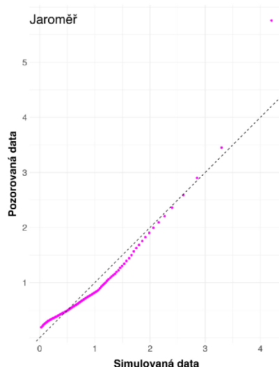
Obrázek 23: Rankitový graf zobrazující srovnání kvantilů měřených a simulovaných dat modelem BILAN na povodí měrné stanice v Maršově.
