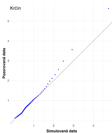
Obrázek 33: Rankitový graf zobrazující srovnání kvantilů měřených a simulovaných dat modelem TUW na povodí měrné stanice v Krčíně.
