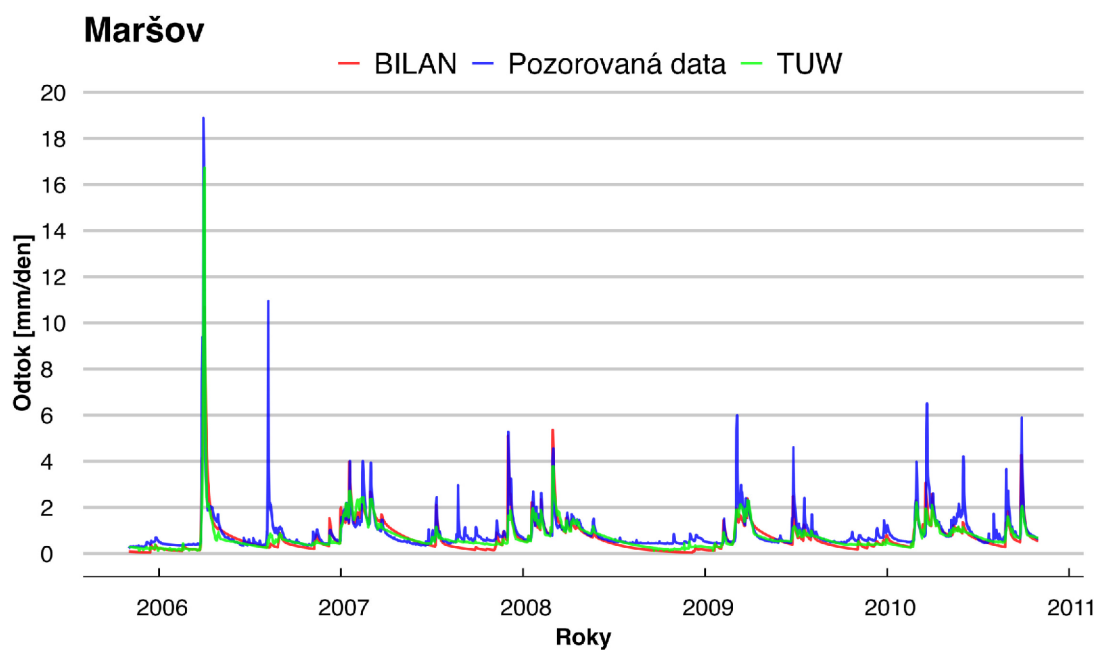
Obrázek 38: Časové řady pozorovaného a simulovaného odtoku na povodí měrné stanice v Maršově mezi lety 2006 a 2011.
