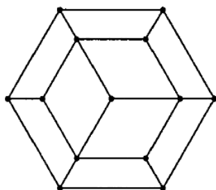
Obr. 2: Kirkmanova plástev [45]
