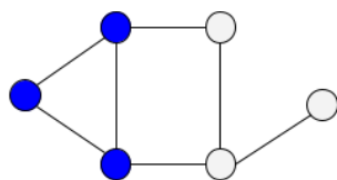
Obr. 9: Graf kliky
