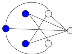
Obr. 10: Graf nezávislé množiny
