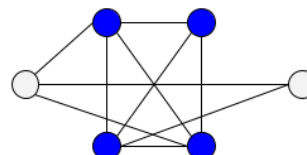
Obr. 12: Graf kliky
