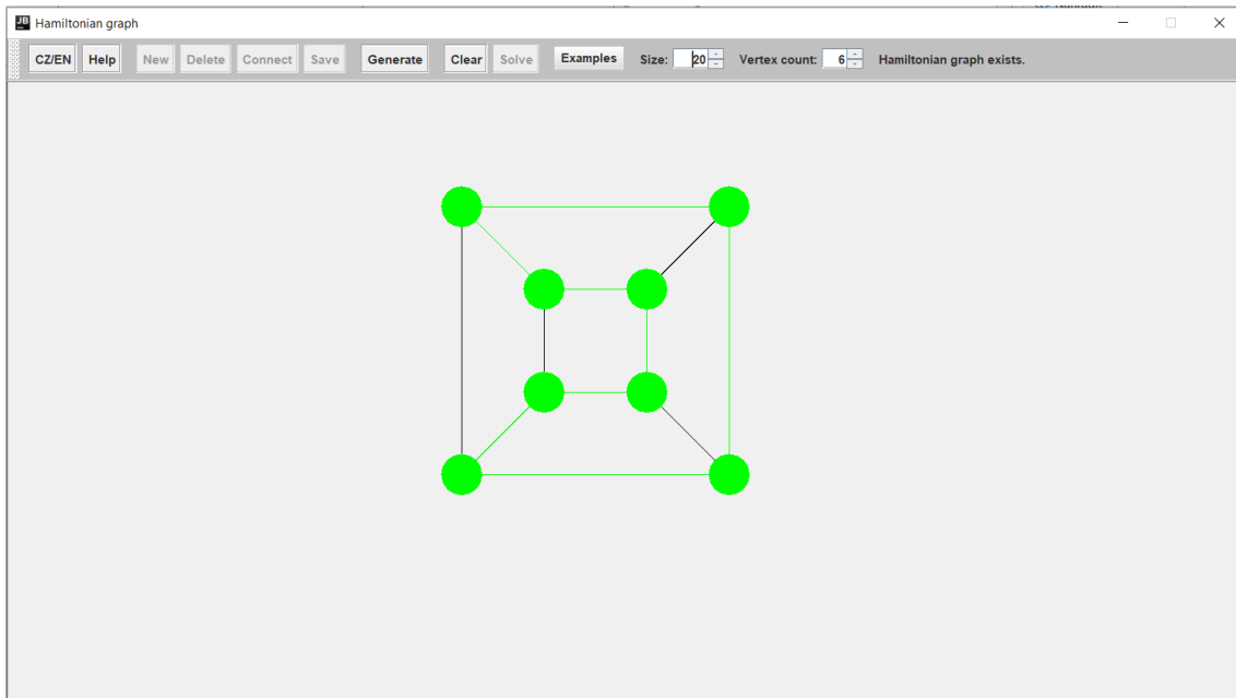
Obr. 22: Okno programu
