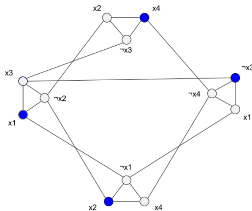
Obr. 15: Vrcholy nezávislé množiny k = 4
