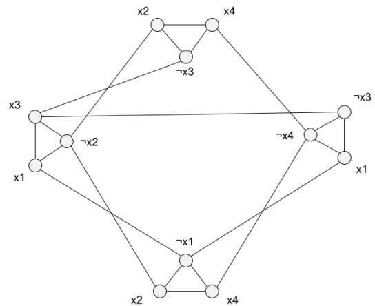
Obr. 14: Spojení klauzulí
