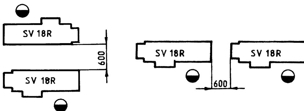
Obr. 1.6 Dvojice soustruhů. [10]
