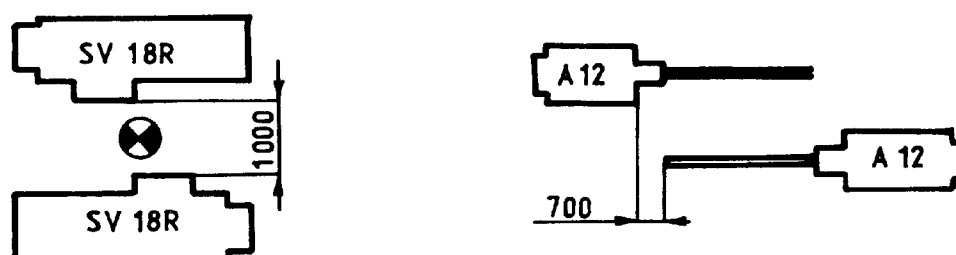
Obr. 1.7 Dvoustrojová obsluha. [10]
