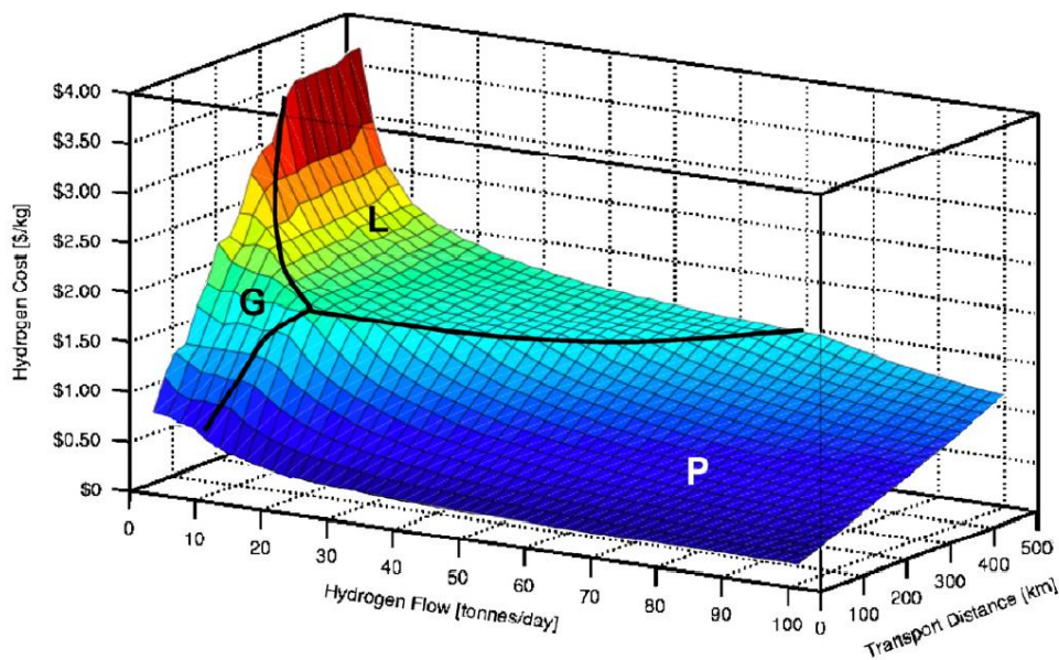
Obr. 7 Nejnižší cena přepravy H_2 jako funkce dopravovaného množství a vzdáleností [21]
