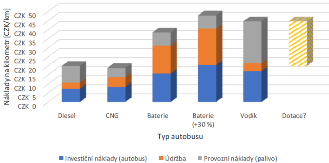
Obr. 17 Přehled nákladů 12m autobusu na kilometr [42]
