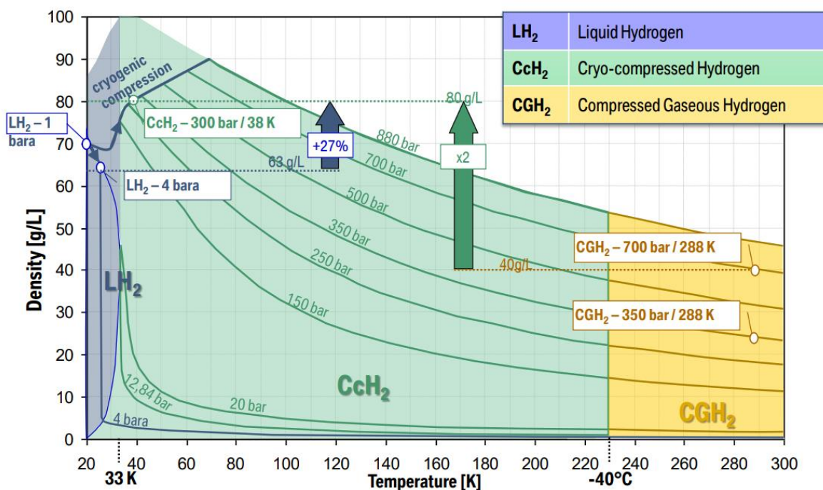
Obr. 6 Porovnání hustoty H 2 při skladování stlačením (CGH 2 ), zkvalněním (LH 2 ) a kryo-kompresí (CcH 2 ) [17]
