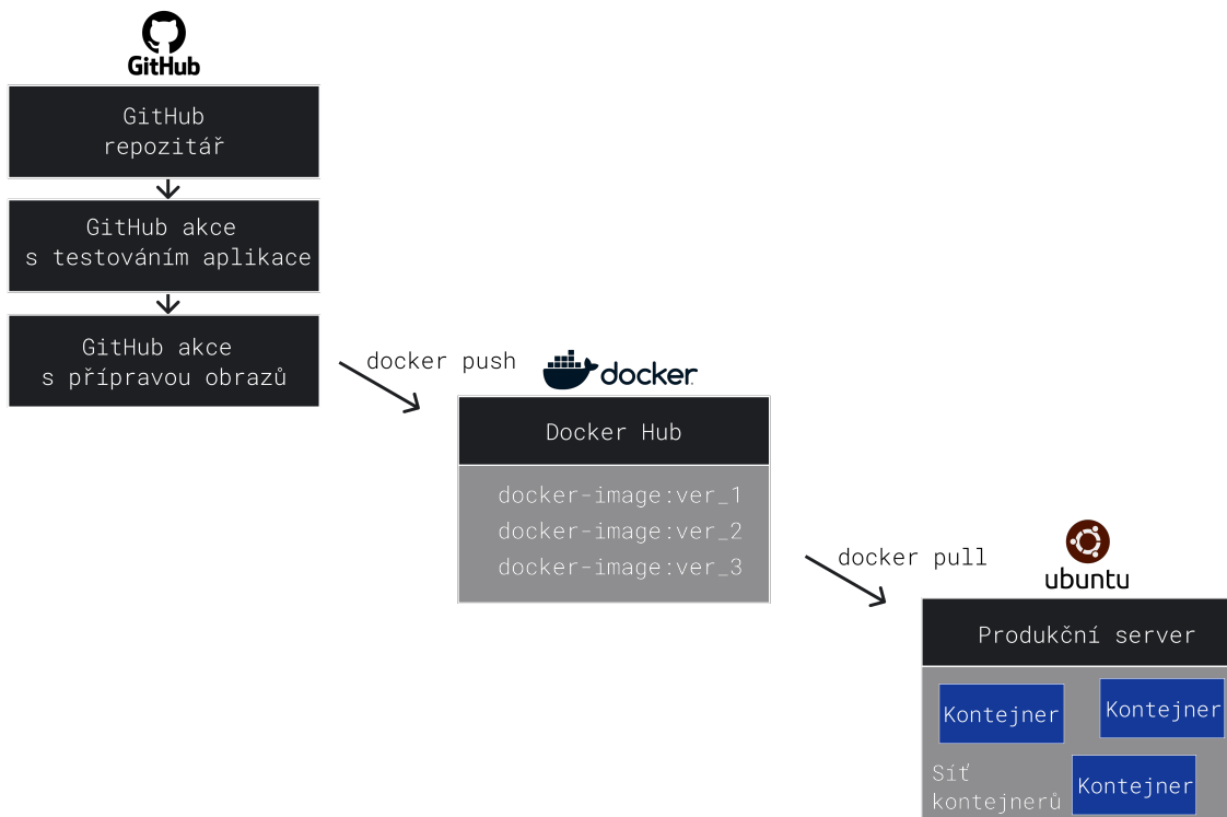
Obr. 3.3: Nasazení aplikace.
