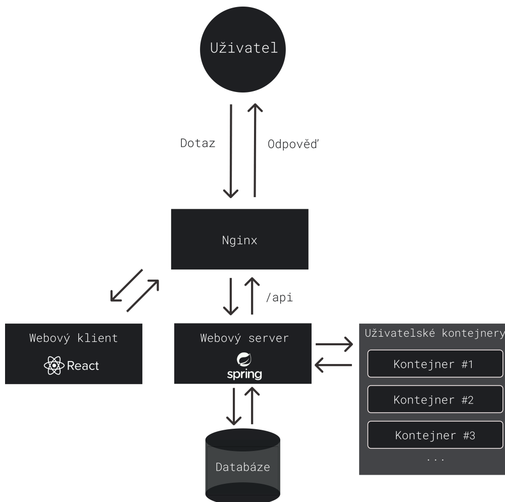
Obr. 2.1: Architektura aplikace.
