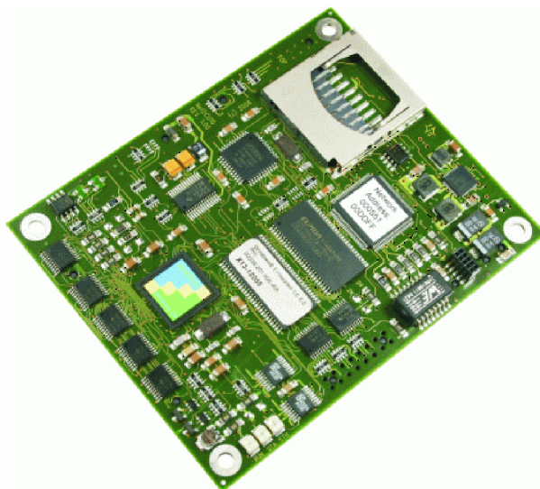
Obrázek 2.6: NetDCU10 bez vývojového kitu s rozhraními
