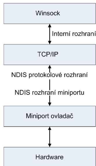
Obrázek 3.13: Architektura NDIS protokolového ovladače
