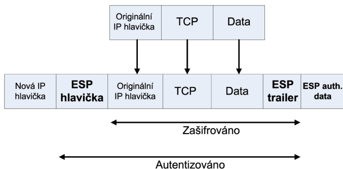
Obrázek 2.5: ESP v transportním a tunelovém režimu
