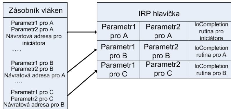
Obrázek 3.8: IRP jako zásobník vláken
