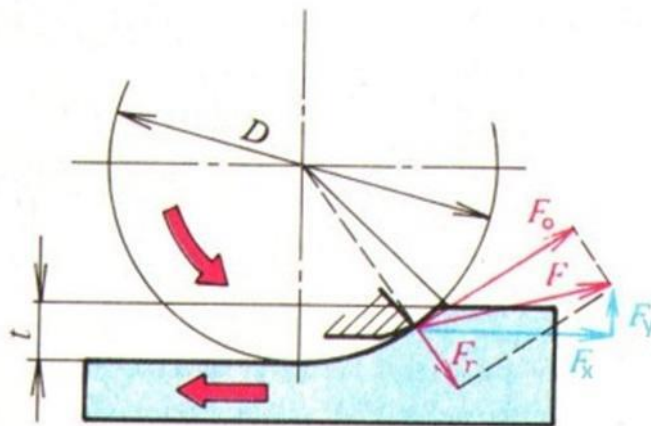
Obr. 3 Nesousledné frézování [3]
