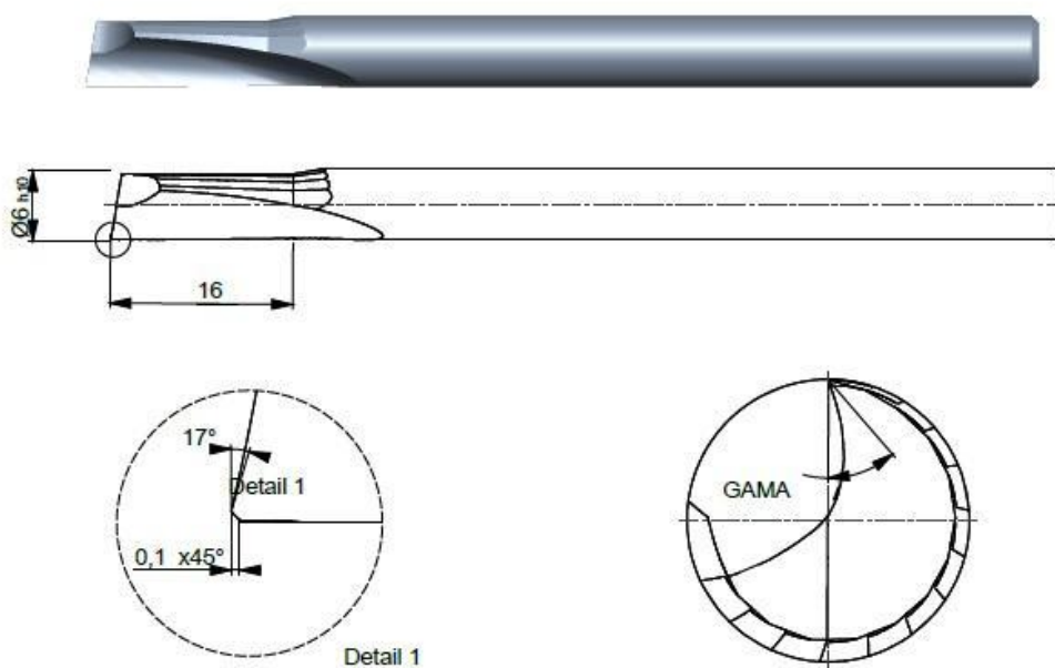
Obr. 21 Obráběcí nástroj
