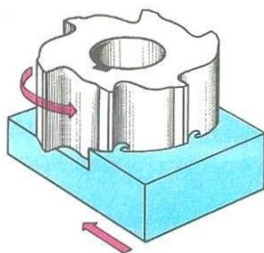
Obr. 1 Čelní frézování [2]
