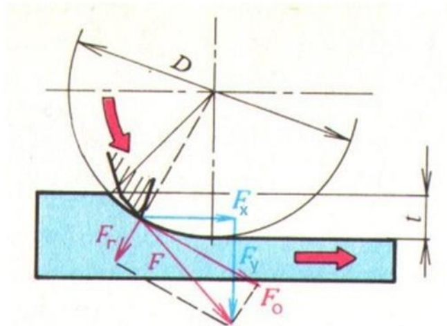
Obr. 2 Sousedné frézování [3]
