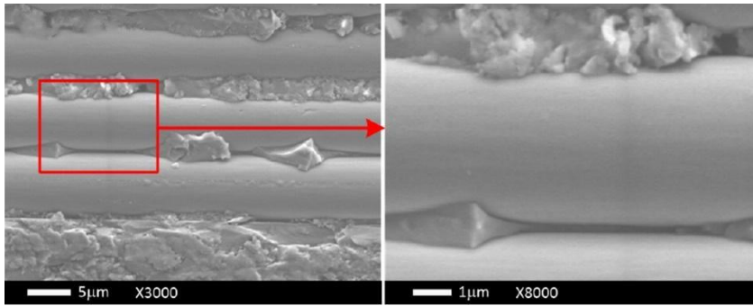
Obr. 12 Oddělení vláken od matrice [19]
