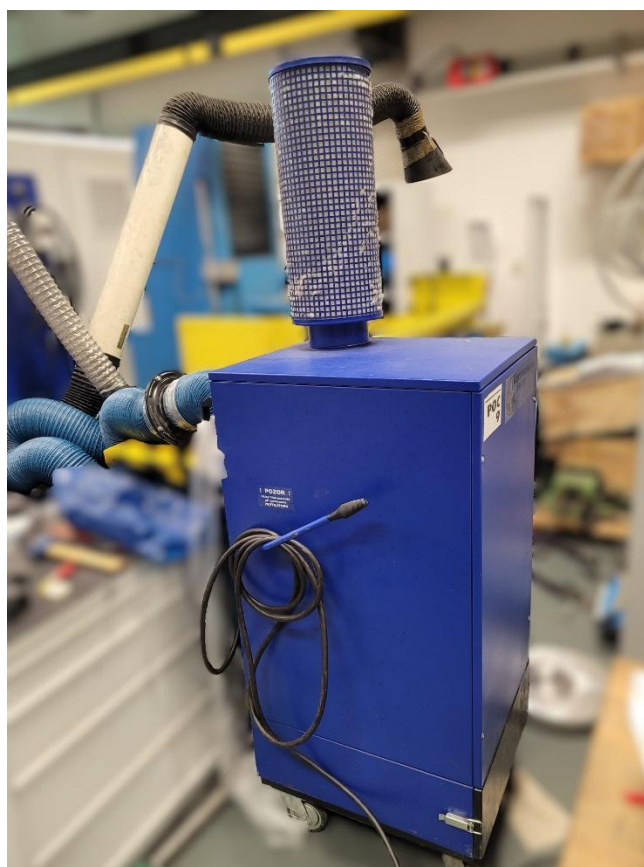
Obr. 20 Odsávací zařízení
