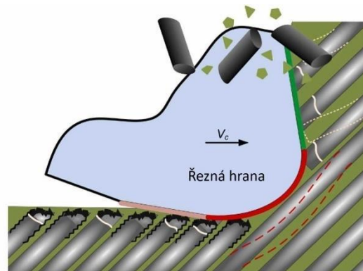
Obr. 8 Úběr materiálu při 45° [16]
