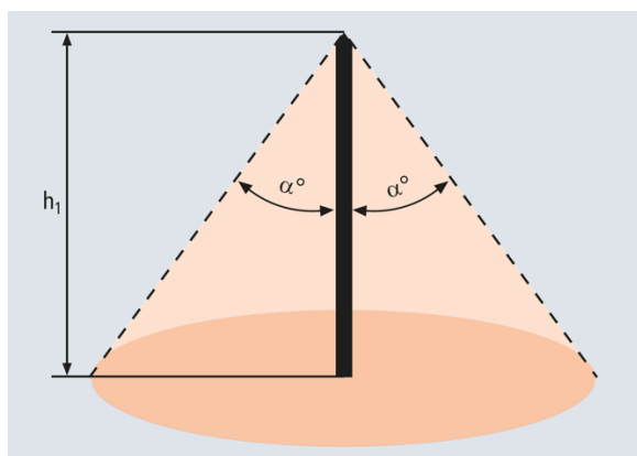
Obrázek č. 8: Ochranný prostor vymezený ochranným úhlem (3)
