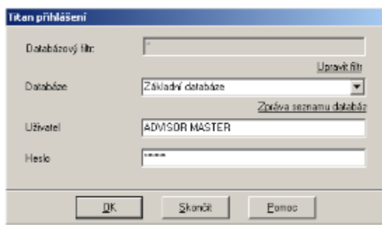
Obrázok 13 Prihlásenie
