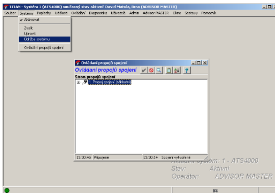
Obrázok 19 Údržba systému
