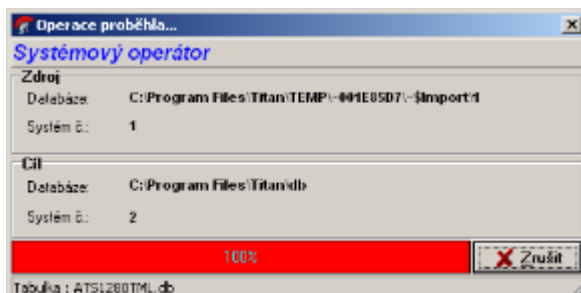
Obrázok 21 Import2
