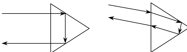
Obrázok 3 Odraž svetla v retroreflexnom prvku
