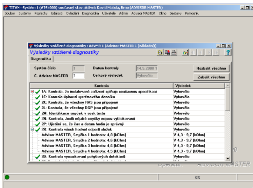
Obrázok 14 Diagnostika
