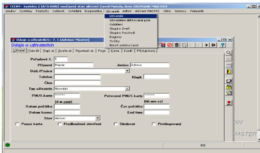
Obrázok 27 Nový užívateľ
