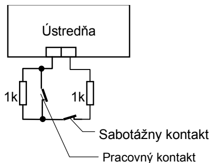
Obrázok 7 Možné zapojenie slučky vyvažovanej 2 odpormi
