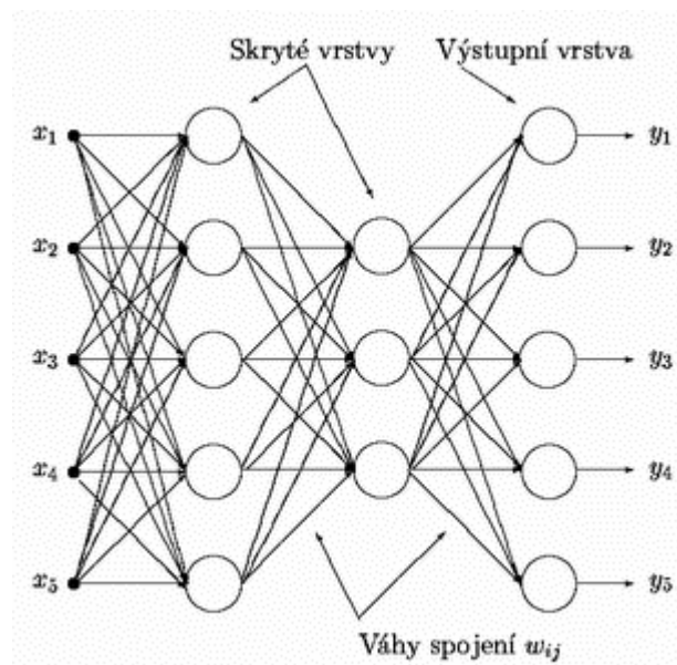
Obrázek 5-5 Topologie vícevrstvé neuronové sítě [2].
