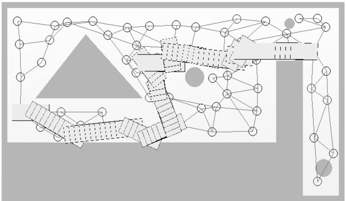
Obrázek 7-9 Trajektorie robotu
