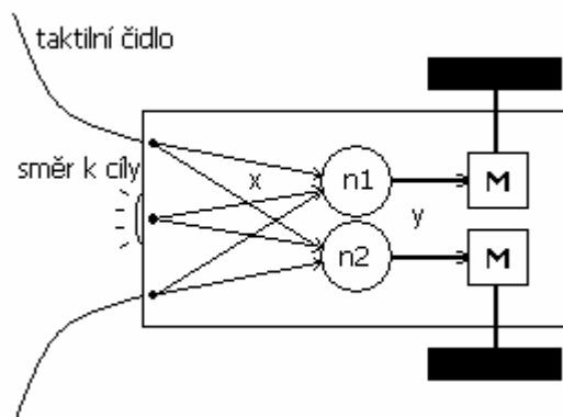
Obrázek 6-1 Robot řízený perceptrony[5].
