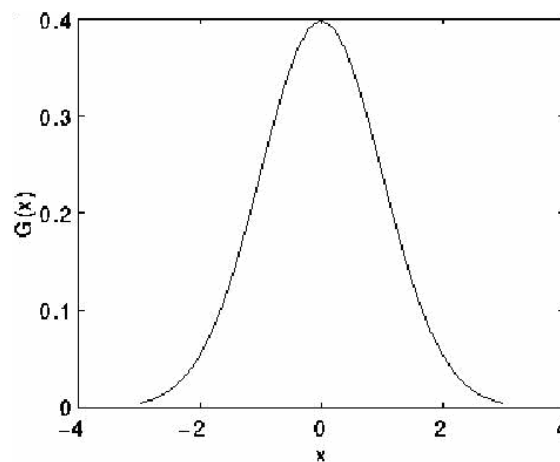
Obrázek 5-8 Gaussova funkce.
