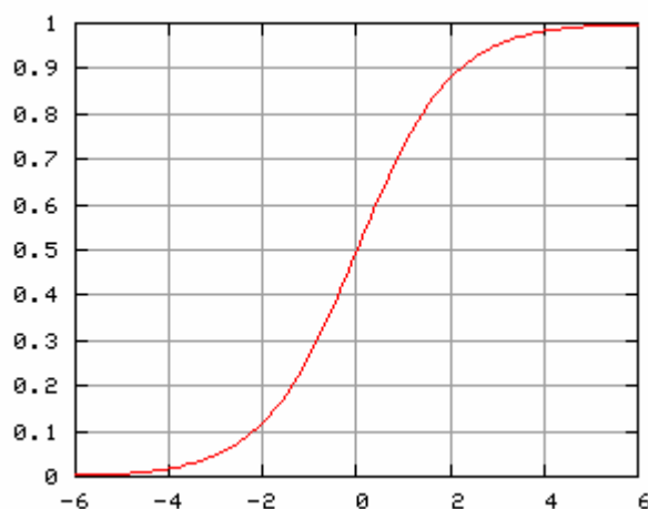
Obrázek 5-4 Sigmoida [8].
