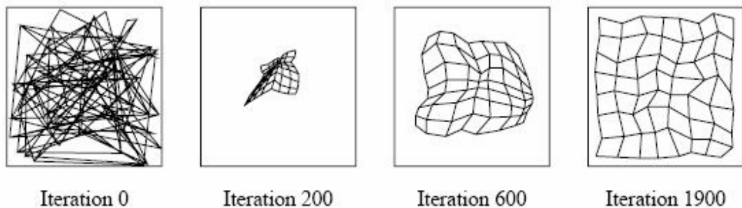
Obrázek 5-10 Postupná adaptace sítě na rovnoměrně rozdělené vstupní data.
