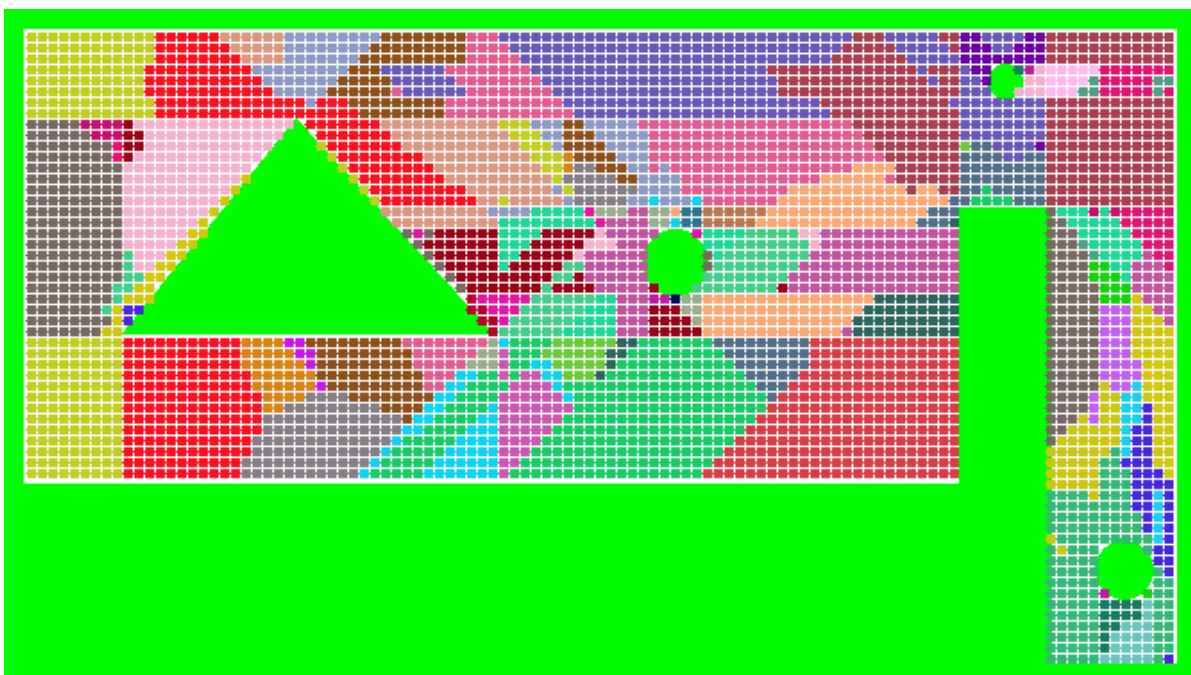
Obrázek 7-5 Rozdělení prostoru do jednotlivých oblastí pomocí SOM.
