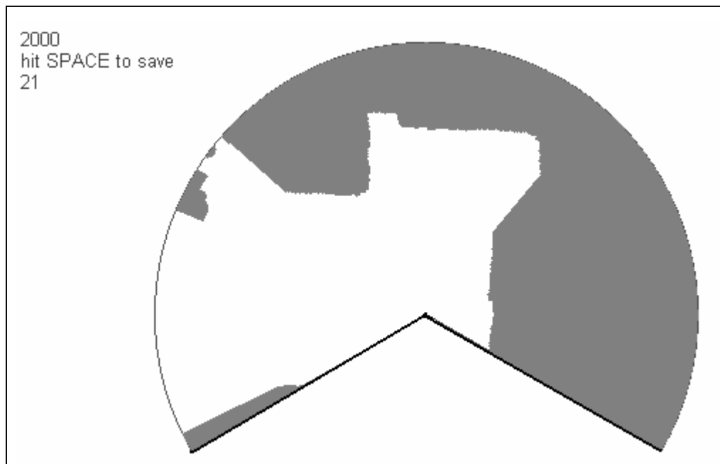
Obrázek 6-5 VizScan.
