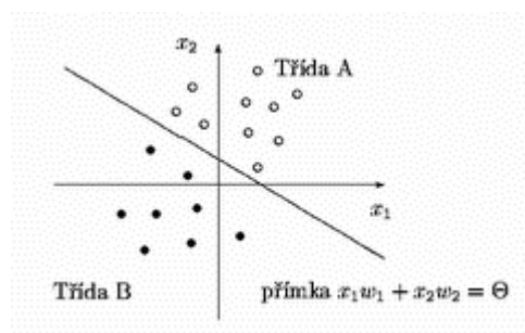
Obrázek 5-2 Rozdělení konfiguračního prostoru jedním perceptronem [2].
