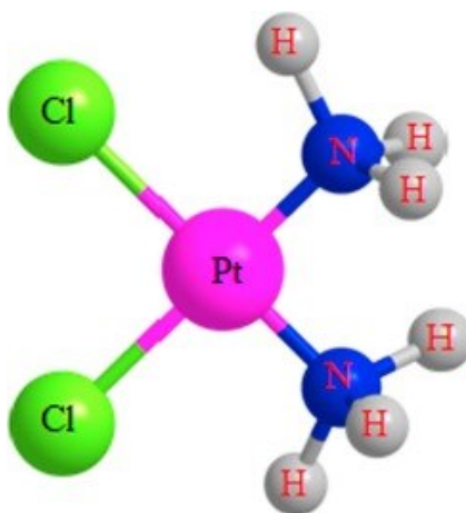
Obrázek 7: Struktura cisplatiny [19].
