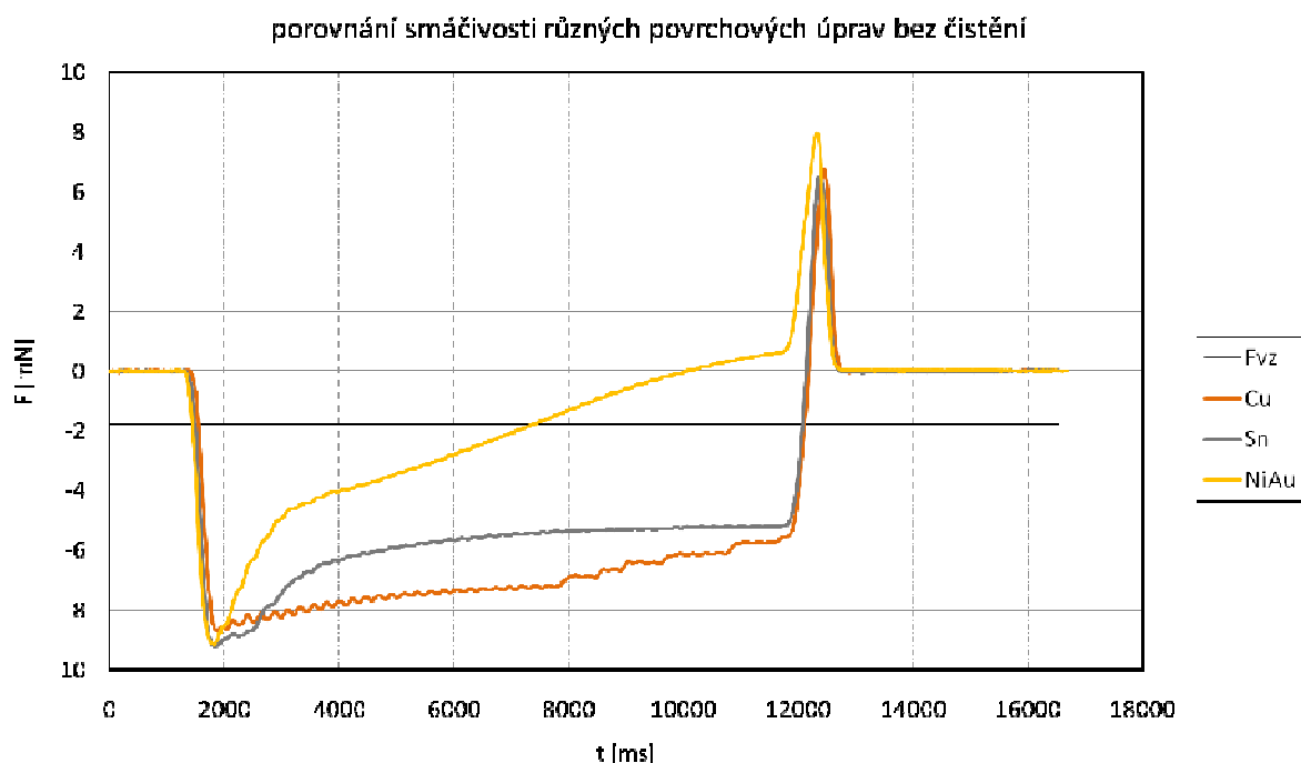
Obrázek 11 Porovnání smáčivosti různých povrchových úprav bez čištění ultrazvukem
