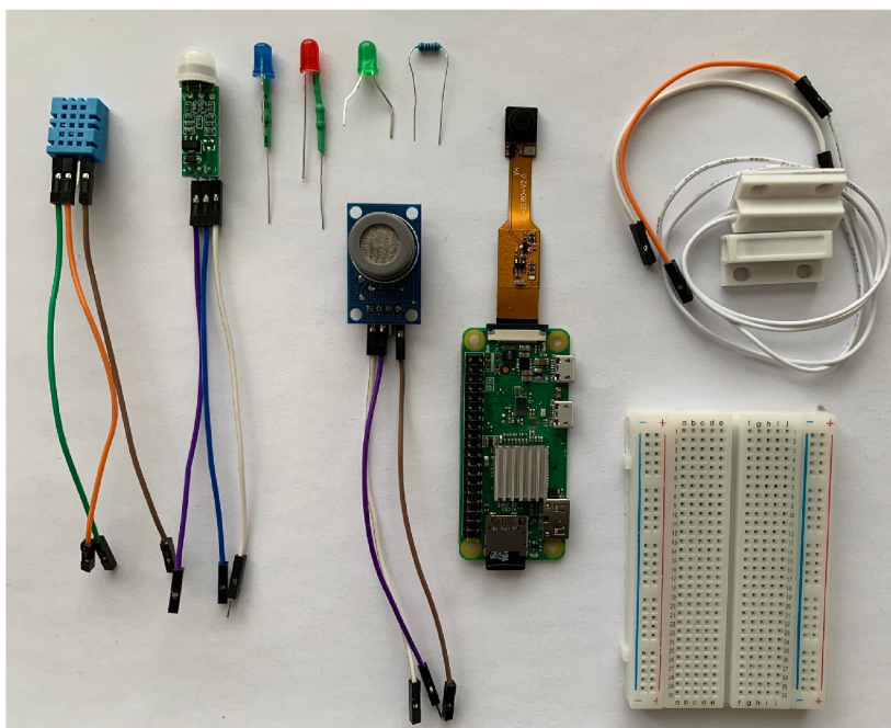
Obrázek 5.2: Použité periferie
