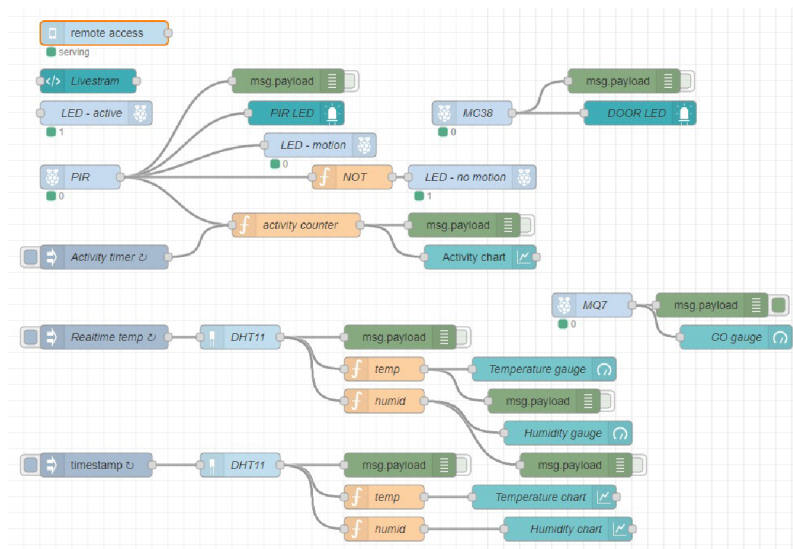
Obrázek 5.11: Kompletní, vytvořený flow diagram v aplikaci Node-RED
