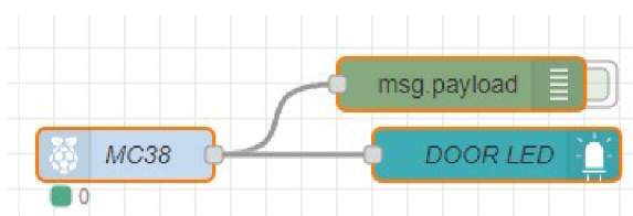
Obrázek 5.8: Logika zapojení sady nodů pro řízení a zobrazování dat ze senzoru MC-38
