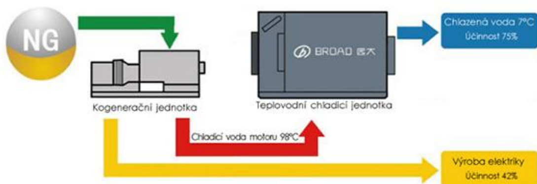
Obrázek 5: Trigenerace
