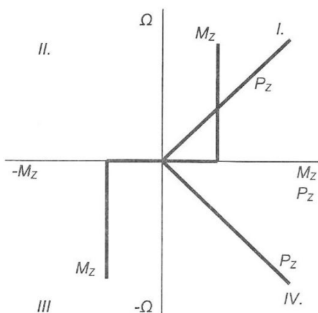
Obr. 1.4 Hoblovková charakteristika [1].
