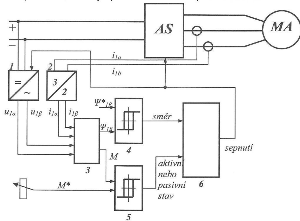
Obr. 2.26 Blokové schéma regulátoru přímého řízení momentu [1].
