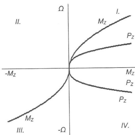
Obr. 1.5 Kalandrová charakteristika [1].
