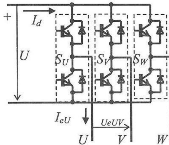
Obr. 2.4 Obvodové schéma třífázového napětového střídače [1].
