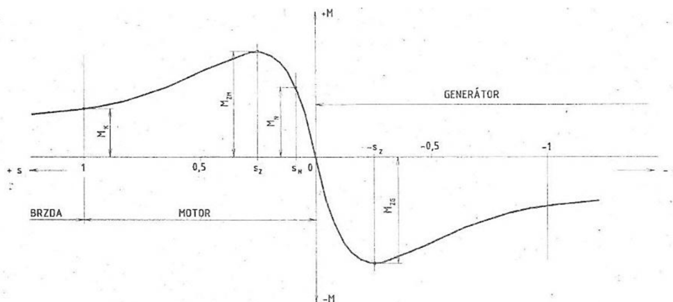
Obr. 2.14 Momentové charakteristika [7].
