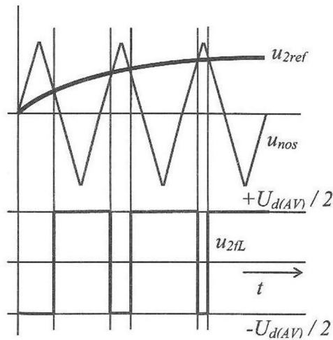
Obr. 2.7 Suboscilační modulace [1].
