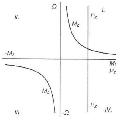
Obr. 1.7 Naviječková charakteristika [1].
