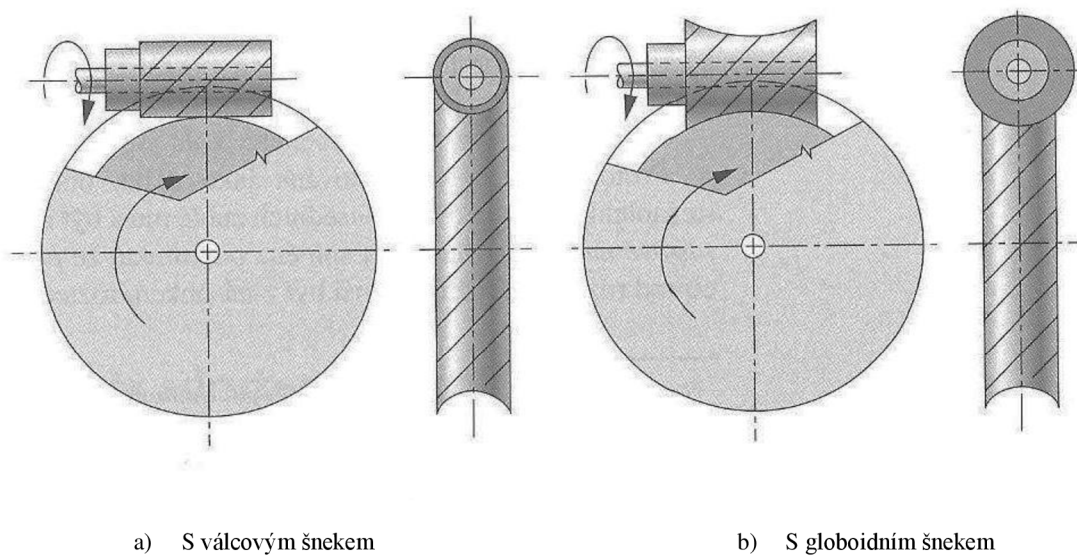
Obr. 3.2 Šnekové soukolí [13].
