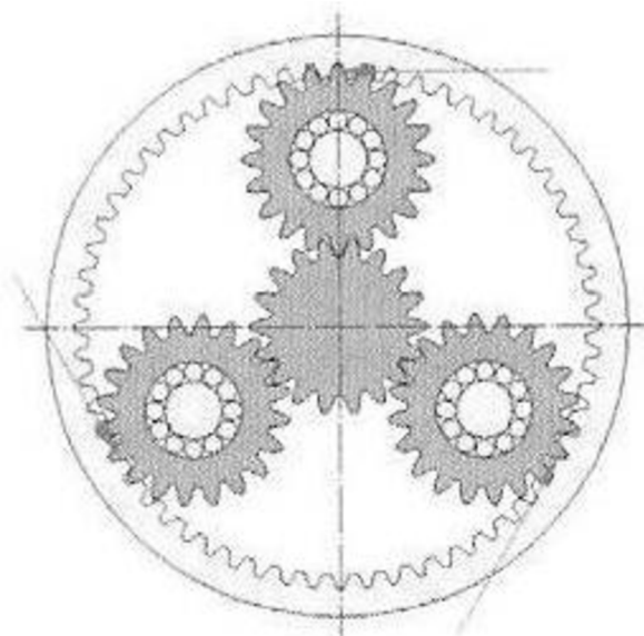
Obr. 3.3 Planetové soukolí [15].
