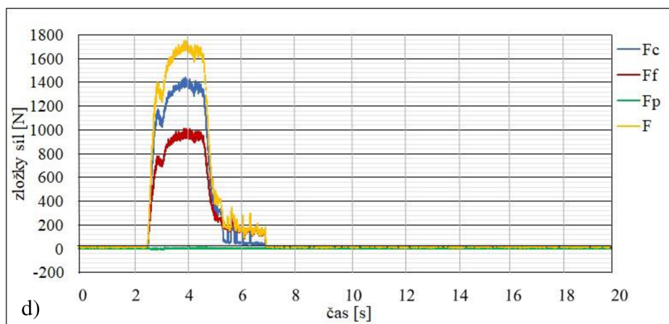
Obr. 4.6 Priebek silových zložiek v_c = 25 \text{ m}\cdot\text{min}^{-1}
