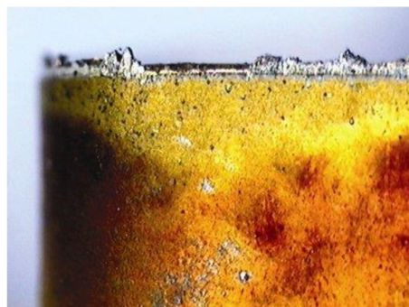
Obr. 3.13 Nárastok na brite [28]
