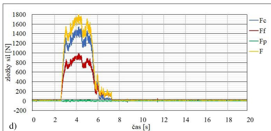
Obr. 4.5 Priebeh silových zložiek v_c = 20 \text{ m}\cdot\text{min}^{-1}
