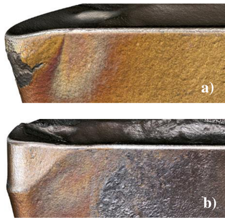
Obr. 3.12 Ostrie britu stlačené (a) a nadvihnuté (b) [5]
