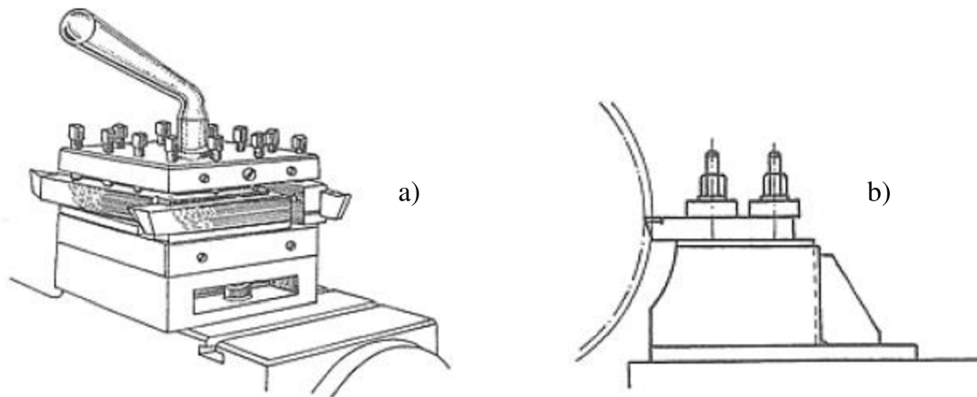
Obr. 2.6 Upnutie nožov za pomoci nožovej hlavy (a) a upínikou (b) [10]
