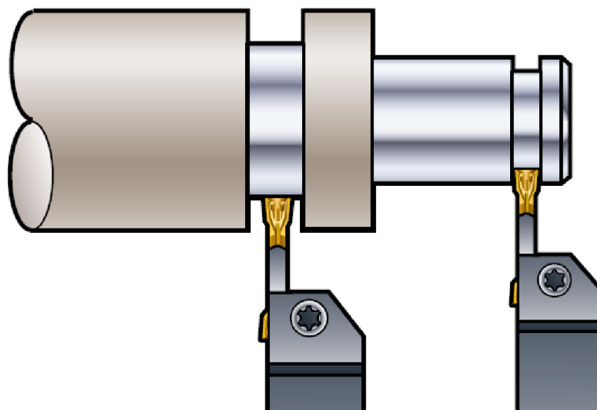
Obr. 1.2 Schéma zapichovania [5]
