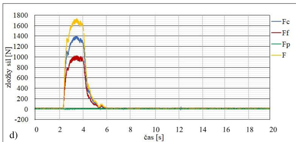
Obr. 4.7 Priebch silových zložiek v_c = 30 \text{ m}\cdot\text{min}^{-1}
