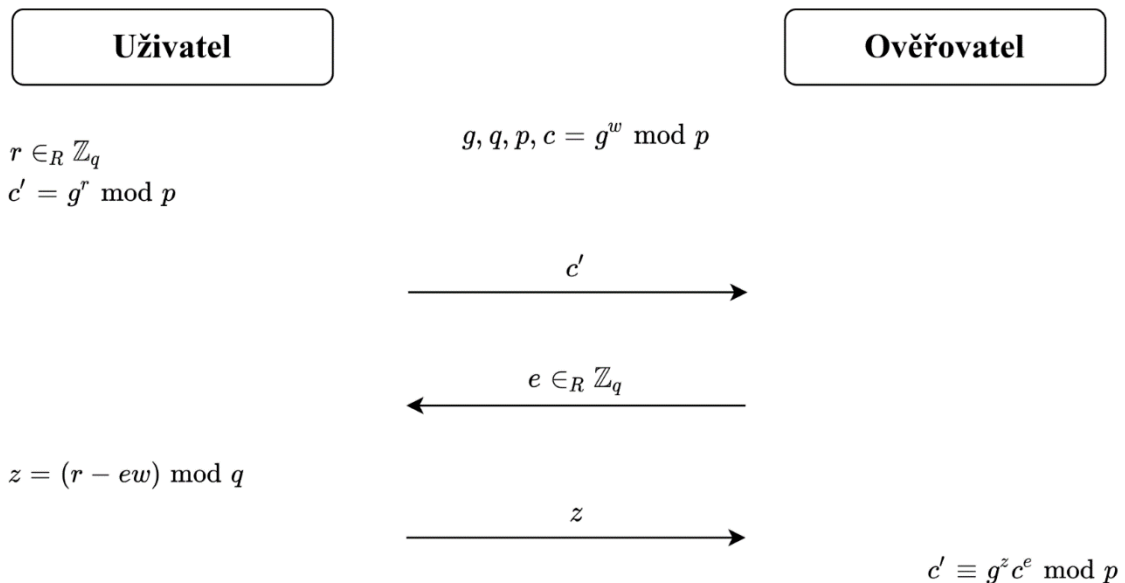
Obr. 1.1: Schnorrův důkaz znalosti diskretního logaritmu
