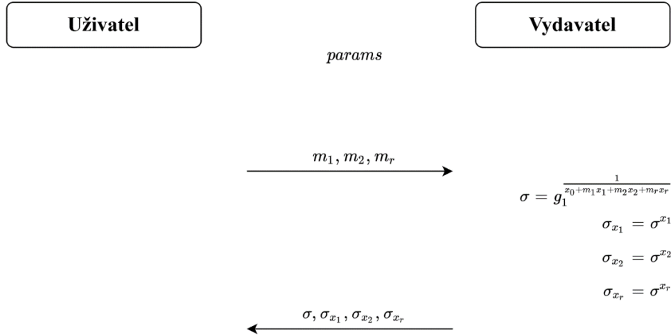
Obr. 1.6: Algoritmus Issue – vydání MAC kódů na atributy
