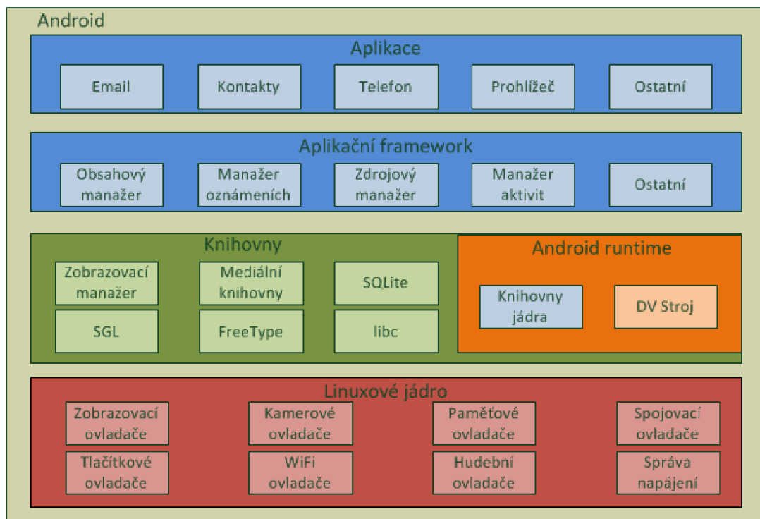
Obr. 5.3: Model vrstev operačního systému Android [15].
