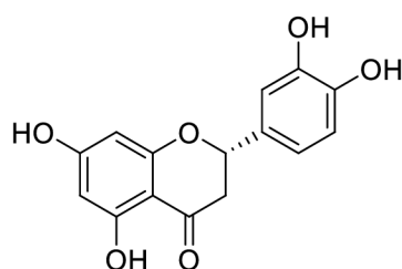
Obrázek 5: Struktura eriodyctiolu
