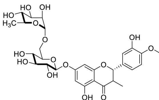
Obrázek 4: Struktura hesperetinu
