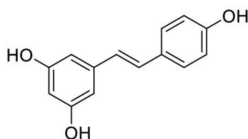
Obrázek 11: Struktura resveratrolu
