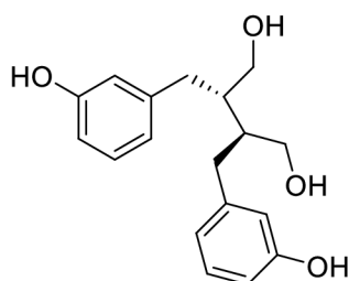
Obrázek 12: Struktura enterodiolu
