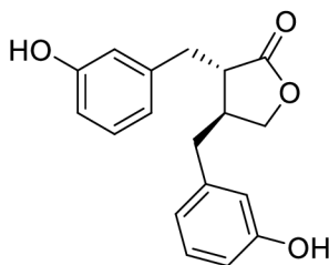
Obrázek 13: Struktura enterolaktonu
