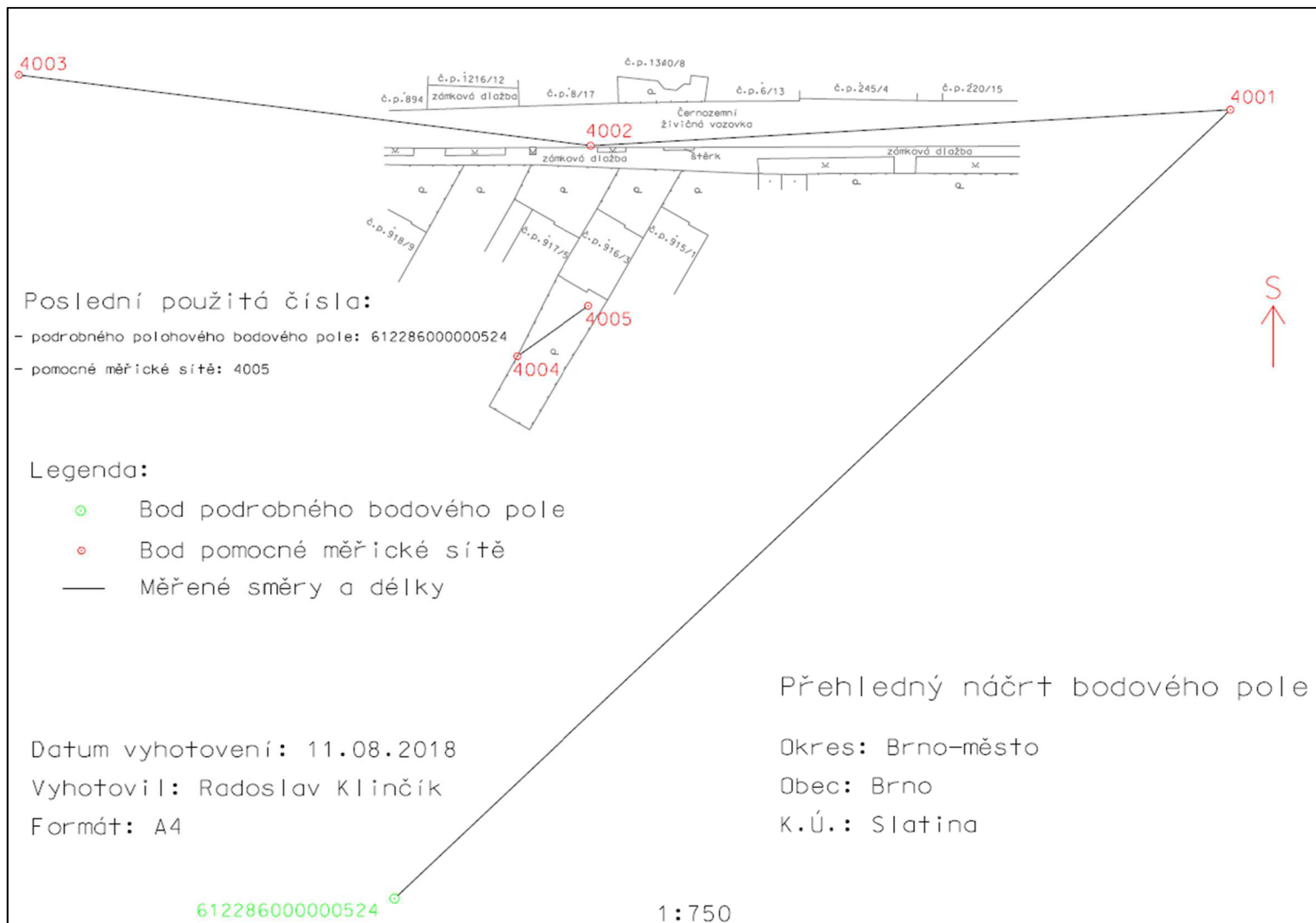
Obr. 8 Ukázka přehledné situace bodového pole
