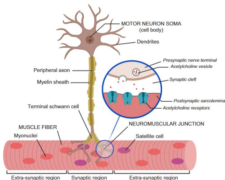
Obrázek 8: Nervosvalová komunikace mezi motoneuronem a svalovým vláknem
