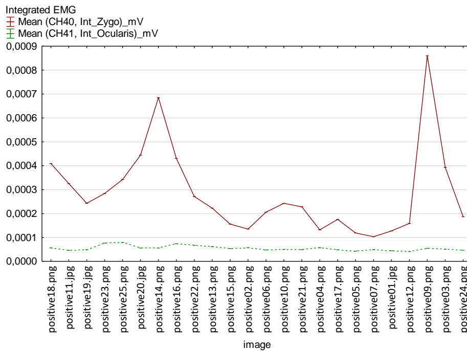
Graf 3: Aktivita svalů úsměvu v reakci na pozitivní podněty zaznamenána jako integrovaný signál EMG
