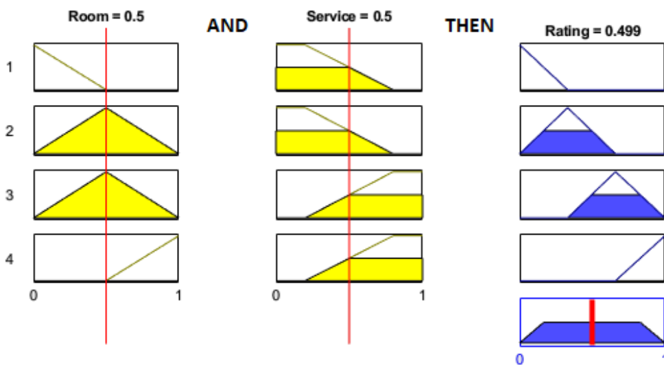
Obrázek 14: Znázornění inference
