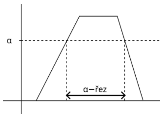
Obrázek 5: \alpha -řez fuzzy množiny
