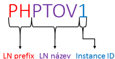
Obrázek 13 - Struktura logického uzlu ochranné funkce
