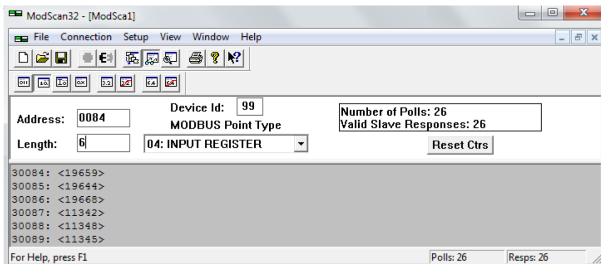
Obrázek 7 - Ukázka vyčítání hodnot pomocí programu ModScan
