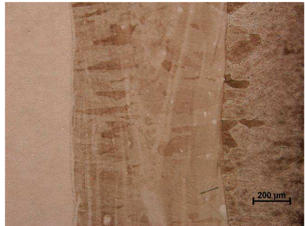
H1, zobrazení střední části svaru
