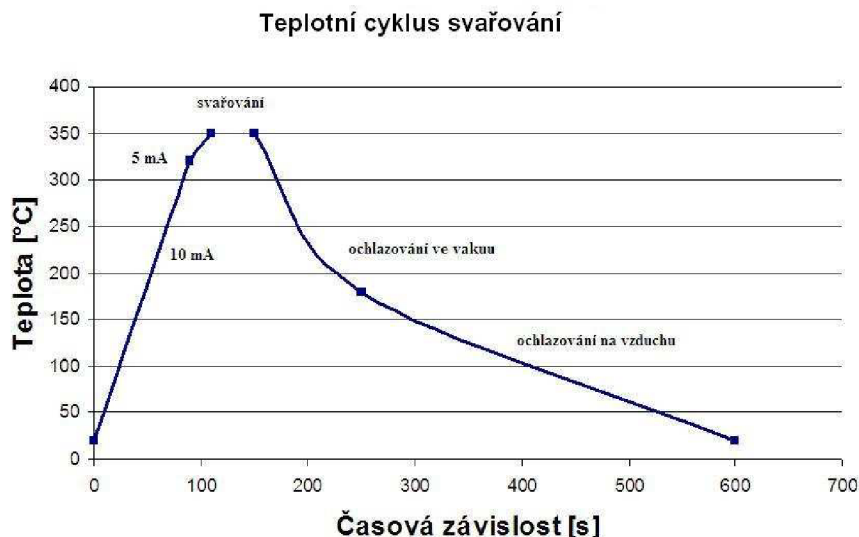
Graf 5: Teplotní cyklus svařování heterogenních feritických svarů
