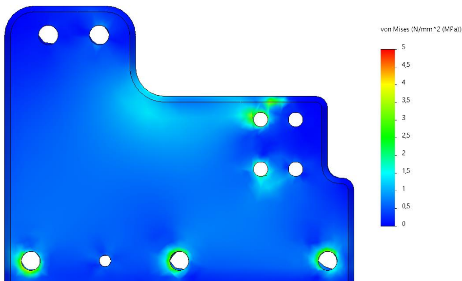
Obrázek 30 Analýza MKP - boční stěna, před odlehčením [25]
