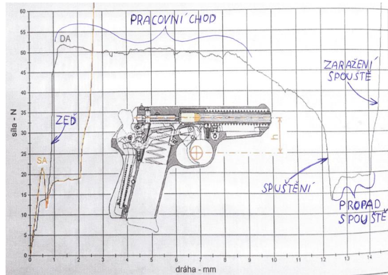
Obrázek 3 Záznam měření spouště ([3], upraveno)
