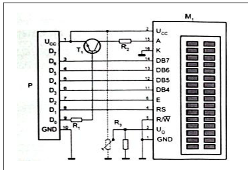
Obr. 5.4.1: Schéma zapojení LCD displeje [16]
