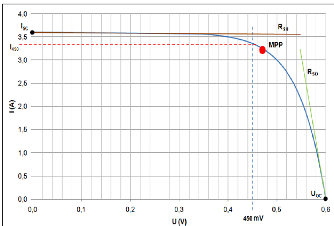
Obr. 3.3.1: VA charakteristika FV článku ( převzato z [10] )
