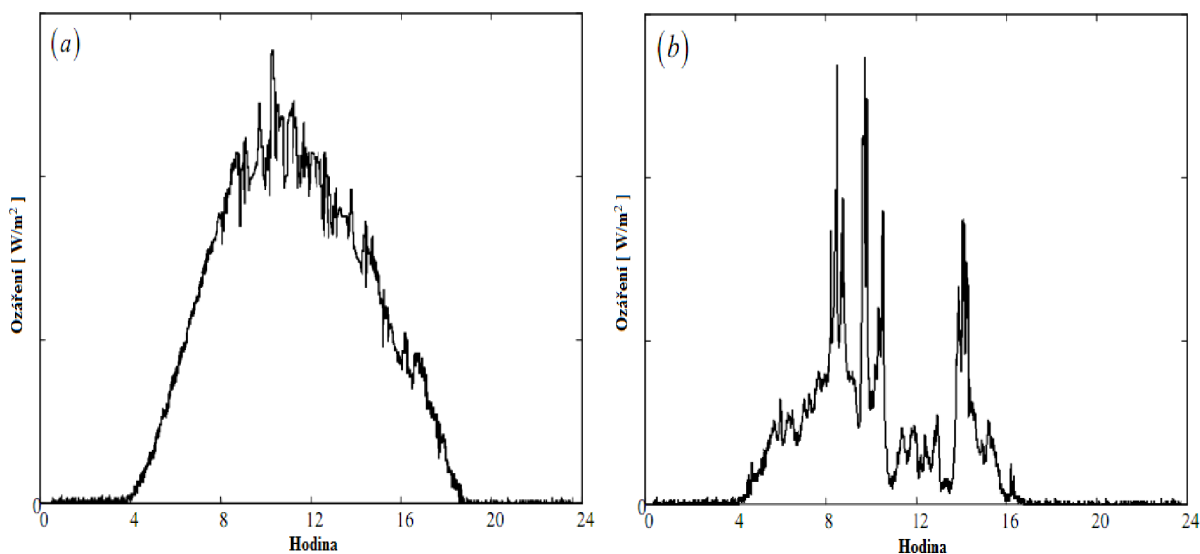
Obrázek 4.1: Průběh intenzity záření během dne. a) slunečný den b) oblačný den [8]
