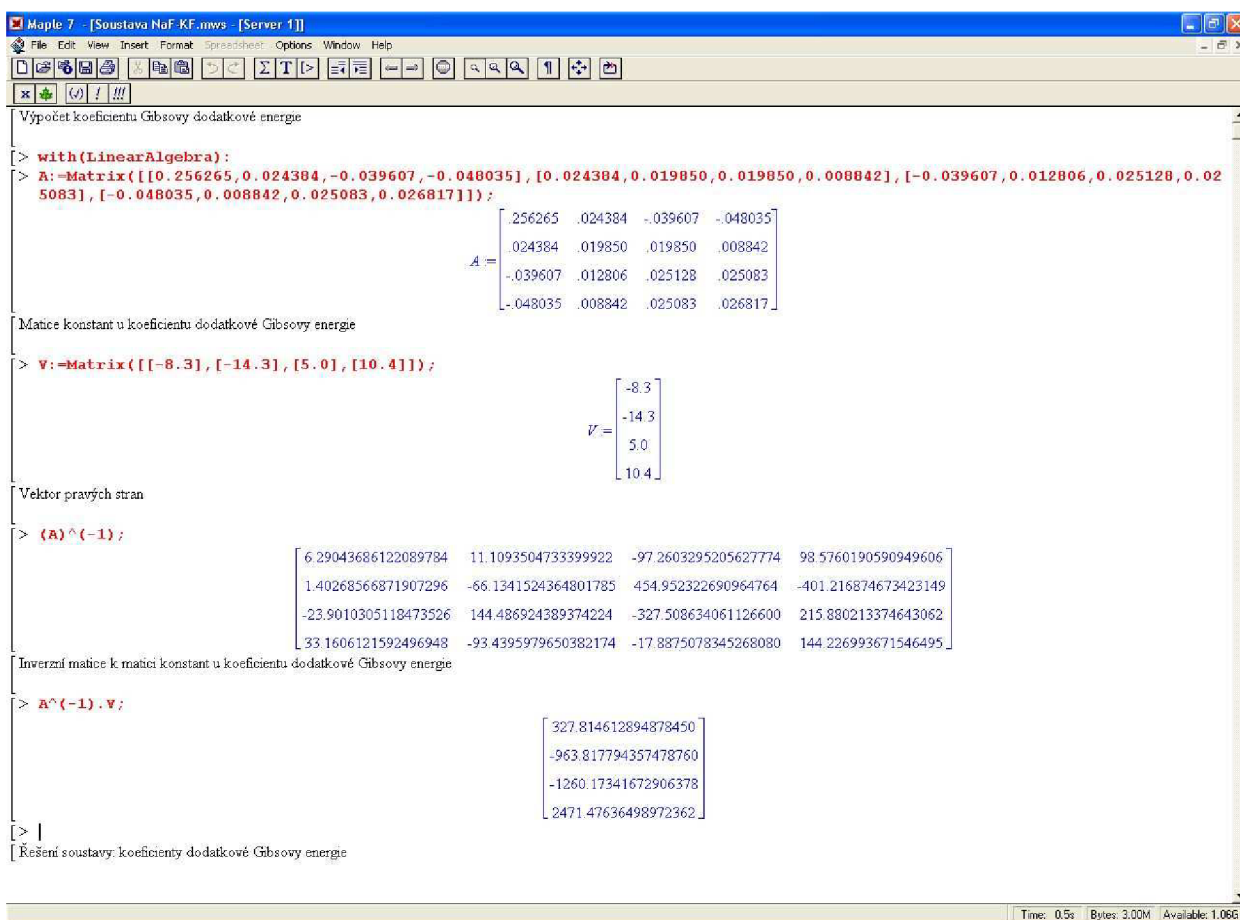
Obr. 5 Výpočet koeficientu polynomu gibbsovy dodatkové energie
