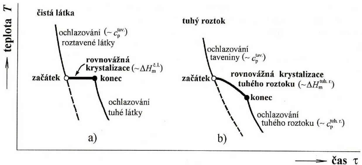
Obr. 3a Ochlazování soustavy s krystalizací čisté látky a tuhého roztoku [9]
