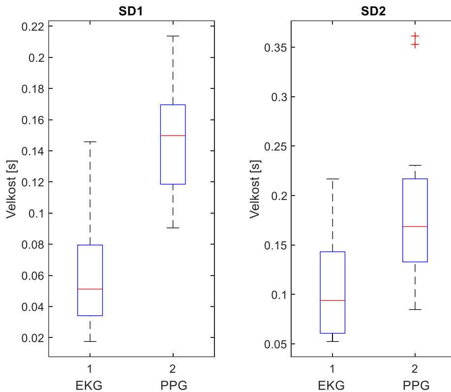
Obr. 6-25 Krabicový graf parametrov SD1 a SD2 pre kľudové záznamy
