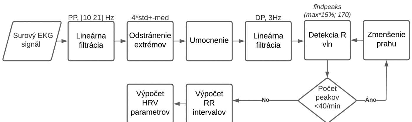
Obr. 6-8 Bloková schéma EKG detektoru
