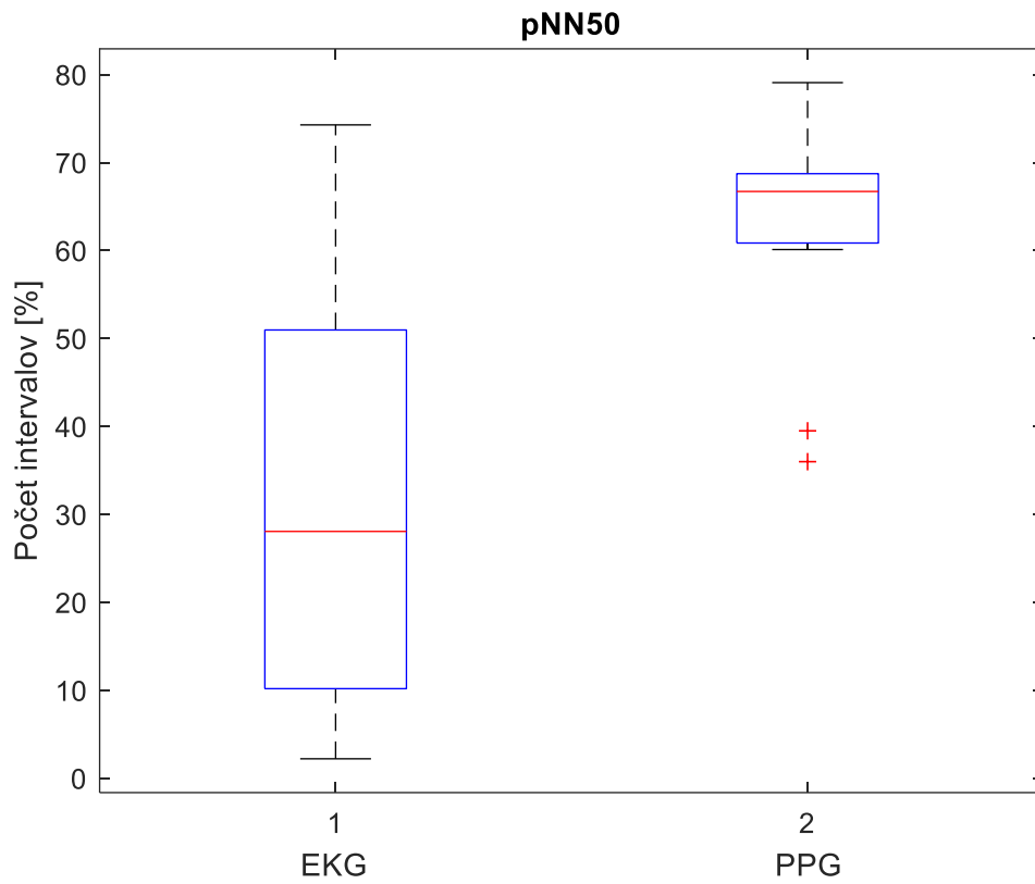
Obr. 6-22 Krabicový graf parametru pNN50 pre kľudové záznamy
