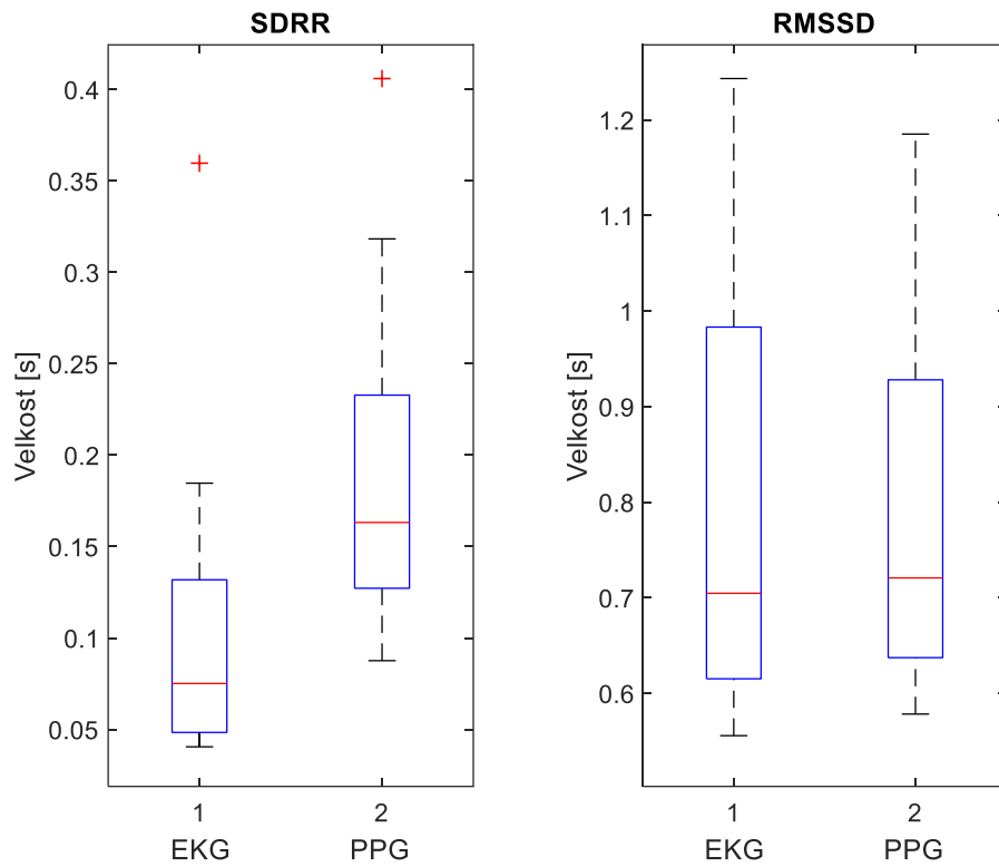
Obr. 6-21 Krabicový graf parametrov SDRR a RMSSD pre kľudové záznamy
