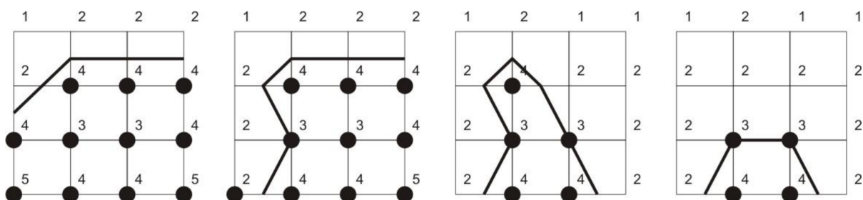
Obrázok 3.6: Príklad hrany mriežky s oboma skalárnymi hodnotami koncových bodov rovných iso-hodnote (3) pretáť nula, raz a dva krát iso-ohraničením. Čierne vrcholy majú skalárnu hodnotu väčšiu alebo rovnú 3 (kladné vrcholy).
