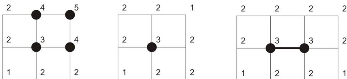
Obrázok 3.5: Príklady hrán dĺžky nula vytvorených MS algoritmom (iso-hodnota 3). Čierne vrcholy majú skalárnu hodnotu väčšiu alebo rovnú 3 (kladné vrcholy). Najľavejší obrázok obsahuje jednu hranu iso-ohraničenia dĺžky nula (z ľavého dolného štvorca mriežky), a prostredný a pravý obrázok obsahujú štyri hrany iso-ohraničenia dĺžky nula. Najpravejší obrázok tiež obsahuje dve nenulové hrany isoohraničenia (z prostredných štvorcov mriežky) ktoré sa priradia na rovnaké hrany mriežky.
