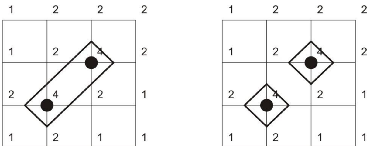
Obrázok 3.7: Typologicky rôzne iso-ohranicenia vytvorene použitím rôznych iso-ohraniceni pre viac významovú konfiguráciu v centrálnej štvorci mriežky.
