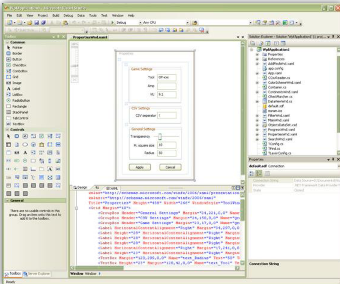
Obrázok 2.1 – Visual Studio 2008
