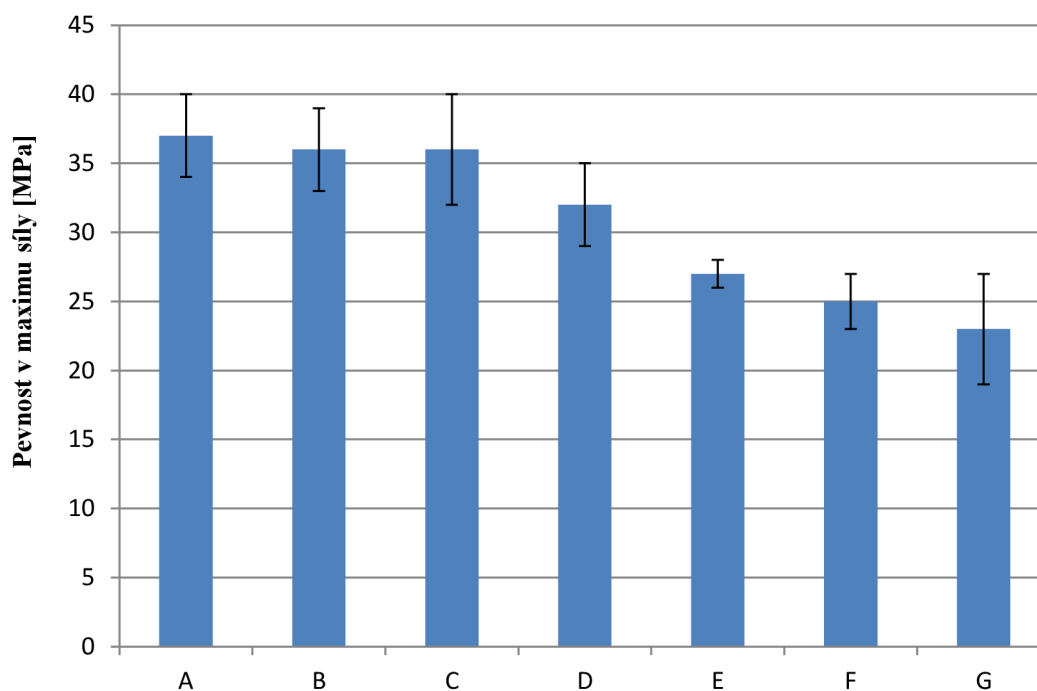
Obr. 23: Graf hodnot pevností v maximu síly pro vzorky ze sady 1
