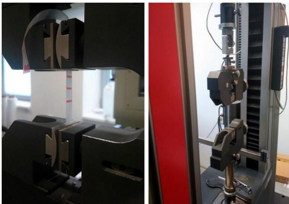
Obr. 11: Vlevo detail upnutí vzorku v čelistech, vpravo fotografie měřicí hlavy a čelistí
