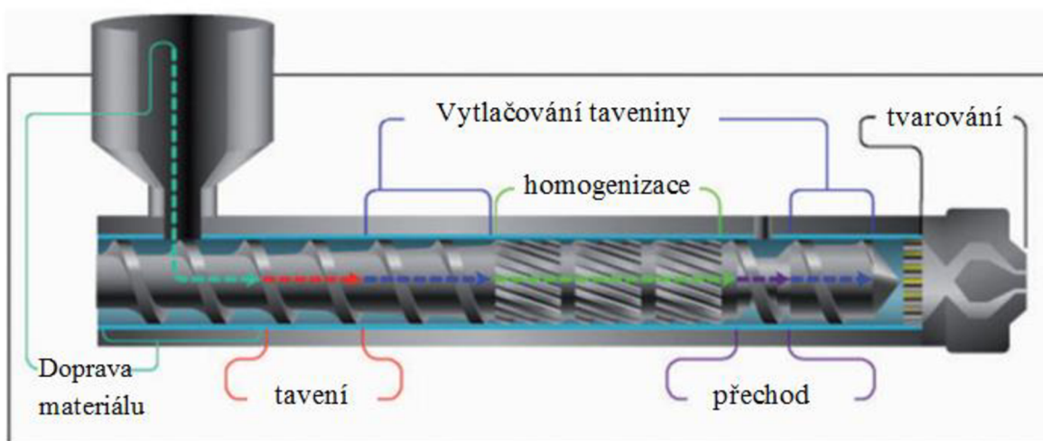
Obr. 4: Funkční zóny extruderu [1]
