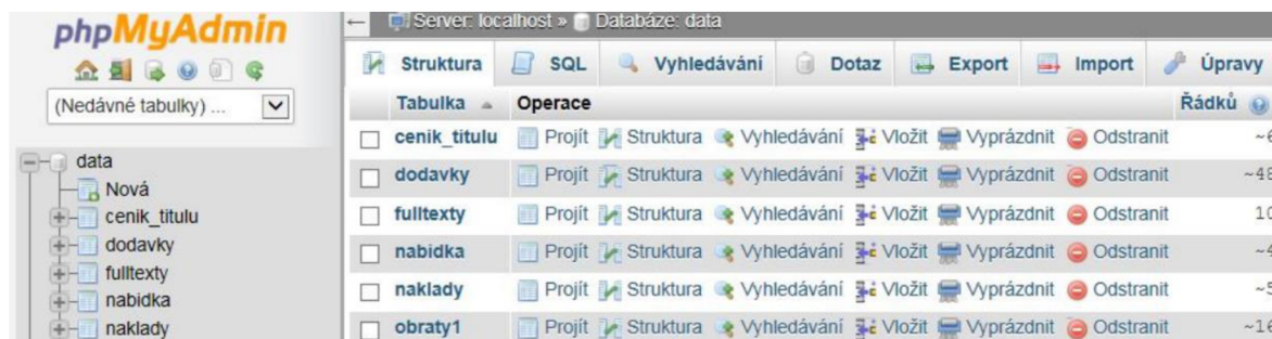
Obrázek 5 - Rozhraní PhpMyAdmin
