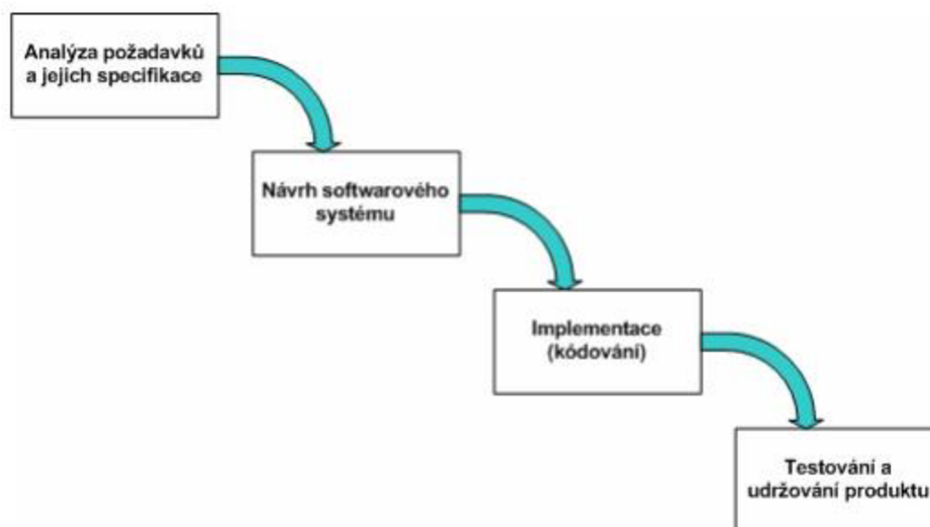
Obrázek 1- Vodopádový model
