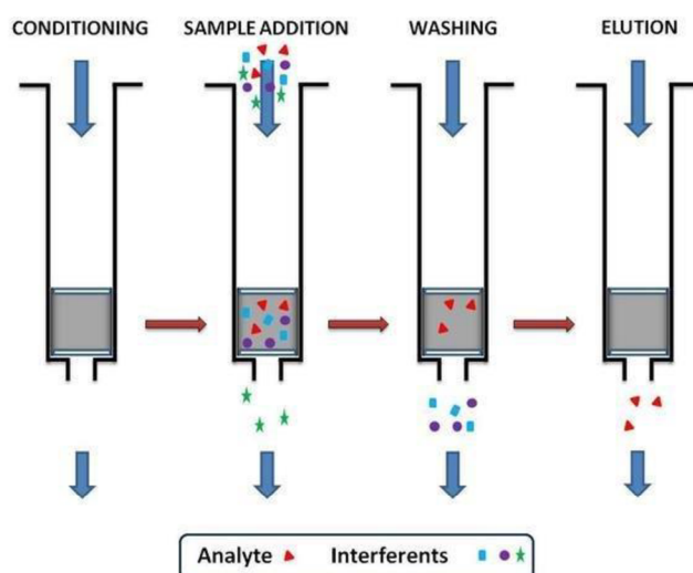
Obrázek 7 – Princip extrakce kapalina – pevná látka (SPE) (Al-Karawi 2016)
