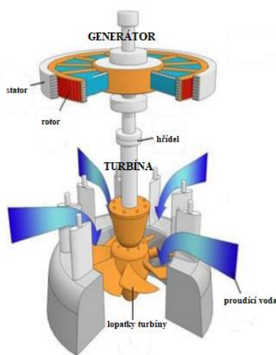
Obrázek 7 Kaplanova turbína
