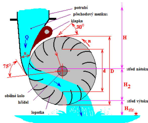
Obrázek 8 Bánkiho turbína
