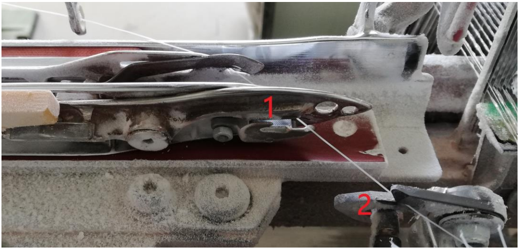
4.5 Odebírání útku jehlou (1) s následným zastřížením nůžkami (2)
