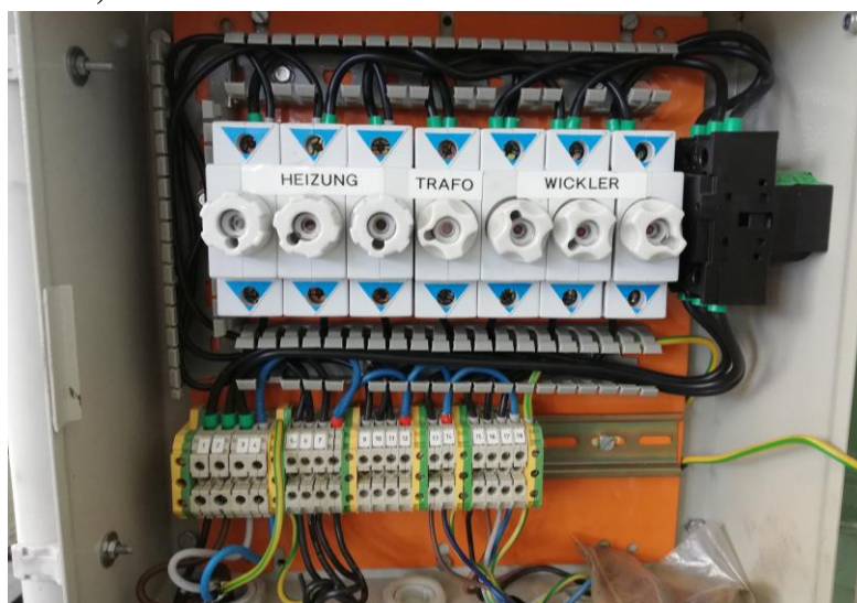
5.3 Přívodní rozváděč tkal. stavu s pojistkami a hl. vypínačem
