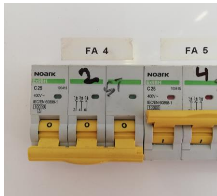
5.1 Znázornění vypnutého jističe v místním rozváděči
