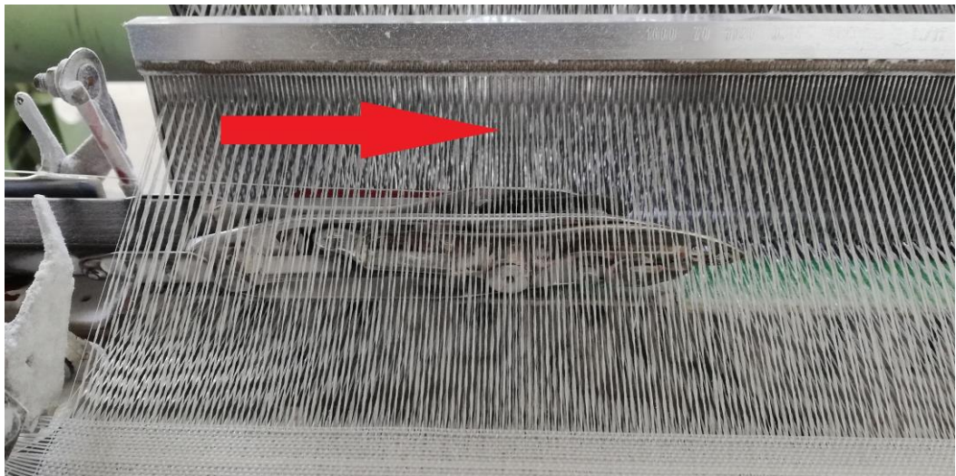
4.6 Zanášení útku jehlou
