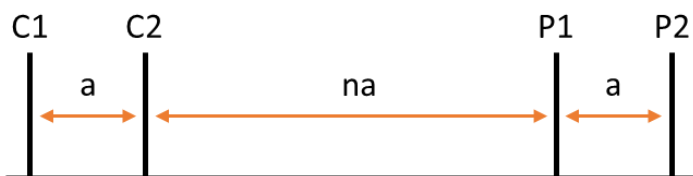
Obr. 7 Dipól – dipól uspořádání elektrod, C1 a C2 – proudové elektrody, P1 a P2 – potenciálové elektrody (upraveno podle Loke 1999). a = vzdálenost, na = násobek vzdálenosti a
