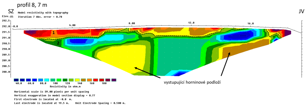
Obr. 18 ERT profily 7 a 8, černou přerušovanou čarou jsou interpretovány předpokládané hranice vrstev podloží a čísla označené domény.
