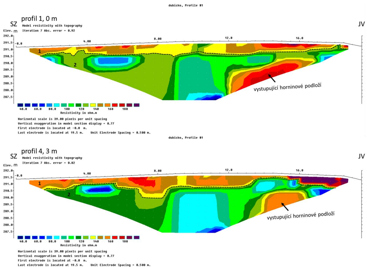
Obr. 17 ERT profily 1 a 4, černou přerušovanou čarou jsou interpretovány předpokládané hranice vrstev podloží a čísly označené domény.
