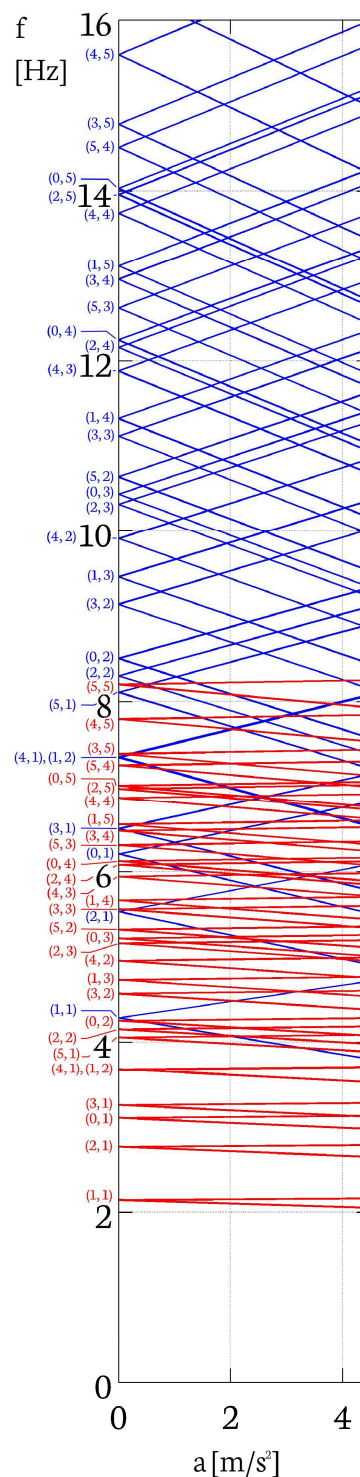
Obrázek 7: Graf hranic nestabilní oblasti některých módů. Červeně jsou módy kmitající izochronně, modře módy kmitající s poloviční frekvencí vzhledem k buzení.
