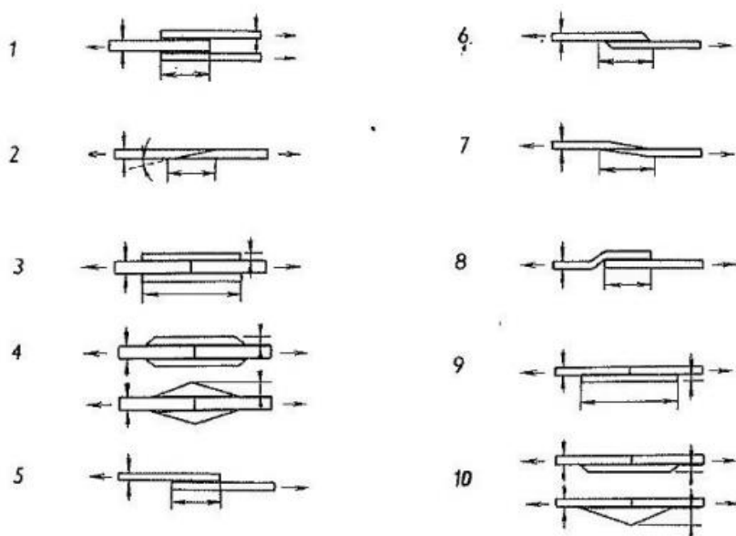
Obrázek 14 Příklad vybraných plochých adhezivních spojů. 1 - dvojitě překlátovaný spoj, 2 - zkosený tupý spoj, 3 - spoj se dvěma příložkami, 4 - spoj se dvěma zkosenými příložkami, 5 - jednoduchý překlátovaný spoj, 6 - jednoduše překlátovaný modifikovaný spoj, 7 - jednoduchý překlátovaný zkosený spoj, 8 - lemový spoj, 9 - spoj s jednou příložkou, 10 - spoj s jednou zkosenou příložkou [11]
