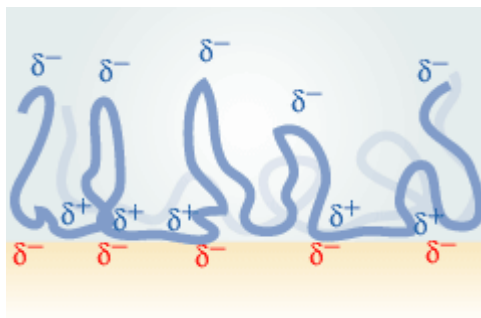
Obrázek 4. Elektrostatická teorie adheze [7]
