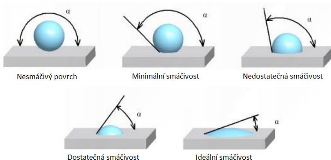
Obrázek 9. Úhel smáčivosti [3]
