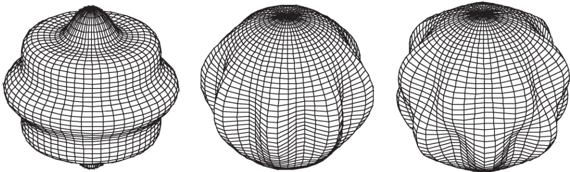
Obr. 1 typy parametrů: zonální (vlevo), sektoriální (uprostřed) a tesserální (vpravo)
