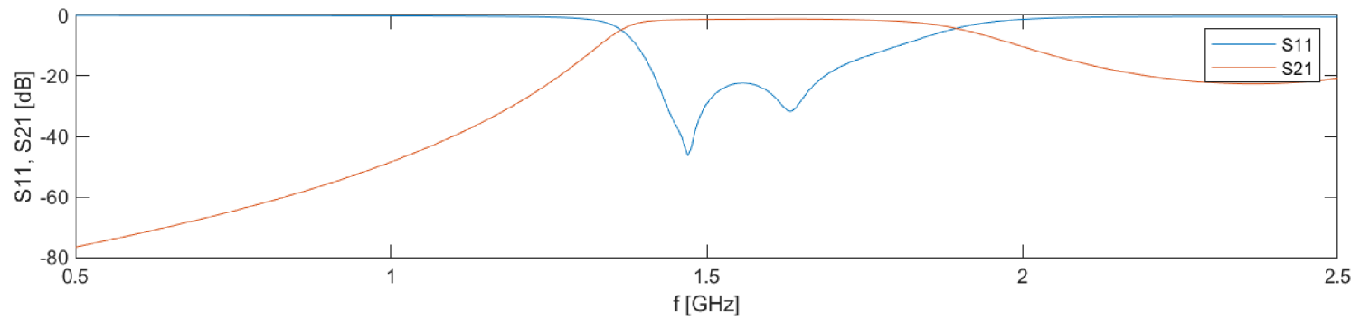
Obr. 3.8: Přenosová charakteristika PP - simulace
