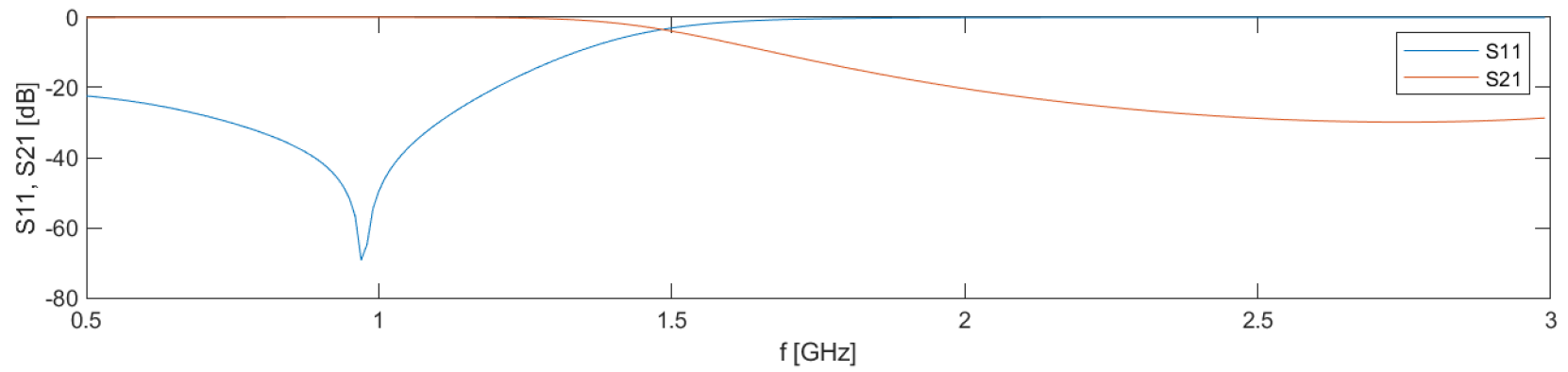
Obr. 3.1: Přenosová charakteristika DP - výstup z aplikace
