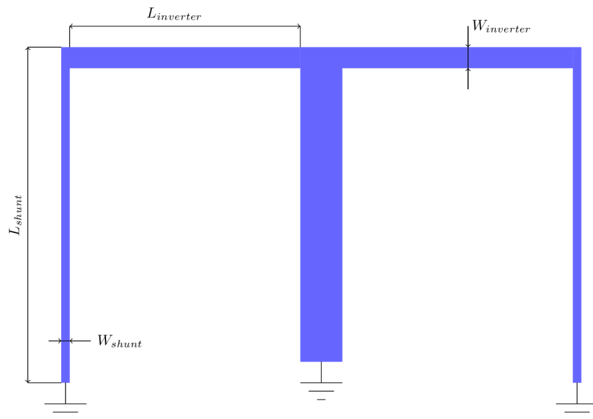
Obr. 2.8: Příklad planární pásmové propusti třetího řádu.
