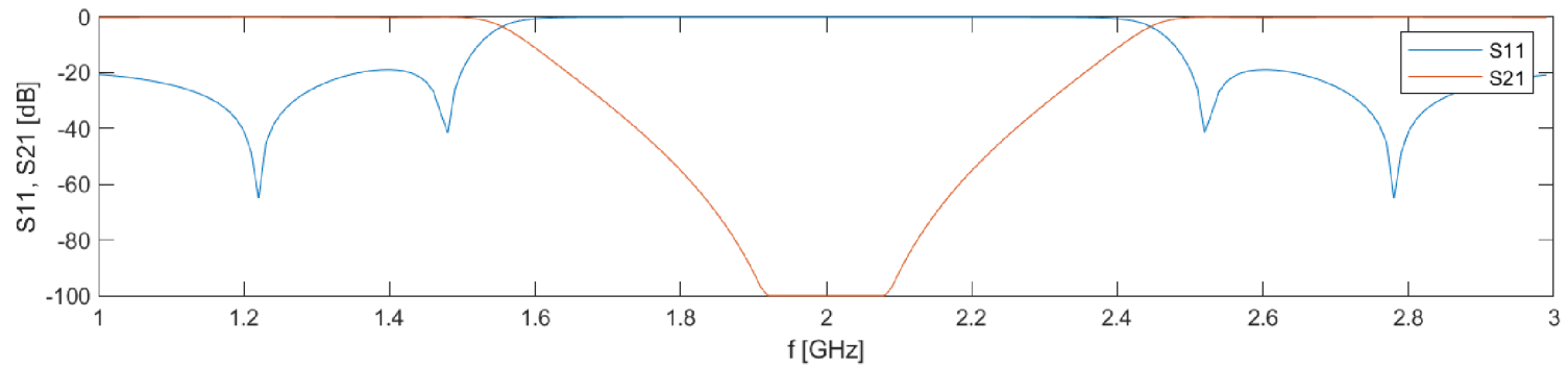
Obr. 3.10: Přenosová charakteristika a vizualizace prototypové PZ
