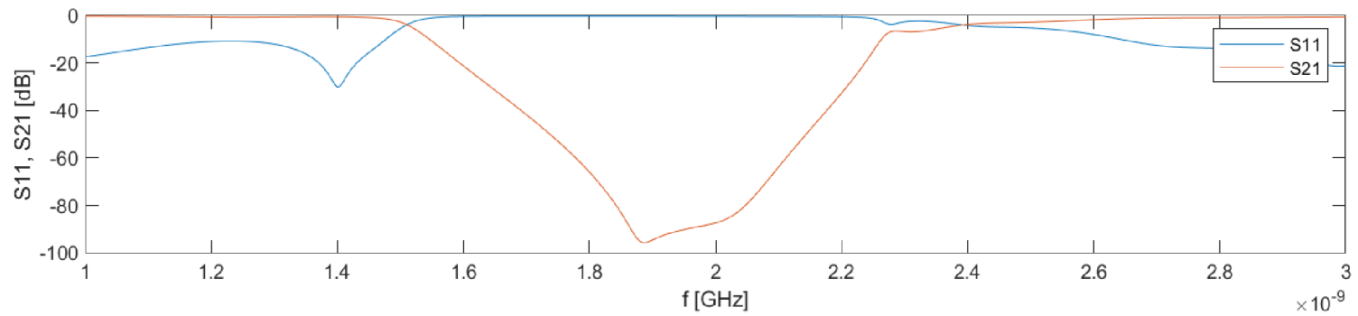
Obr. 3.11: Přenosová charakteristika simulované PZ
