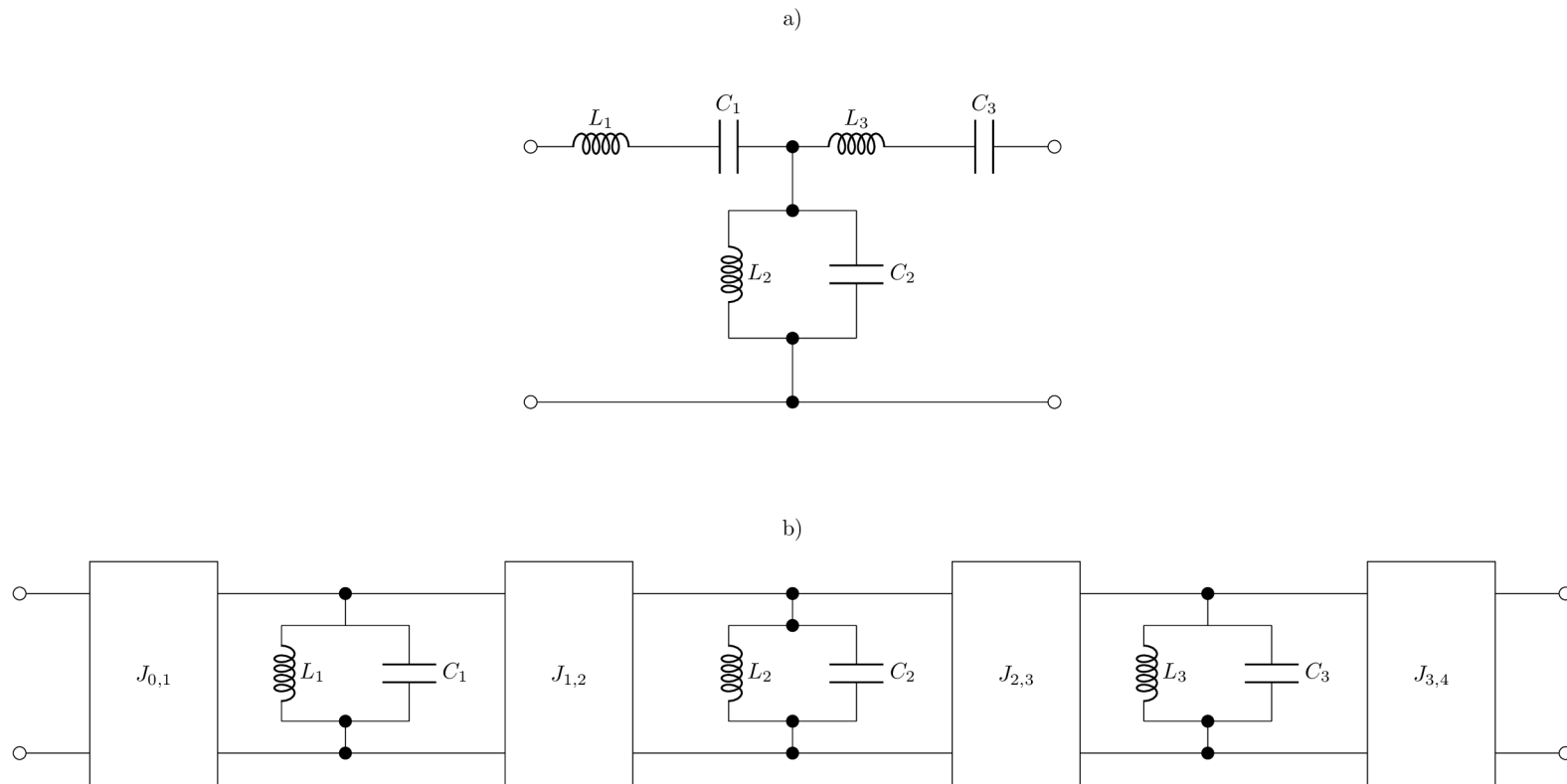
Obr. 2.9: a) Pásmová propust třetího řádu, po transformaci NDP. b) Vložení admitančních invertorů a transformace sériových prvků [1]
