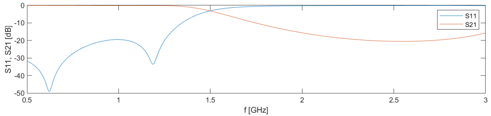
Obr. 3.2: Přenosová charakteristika DP - simulace
