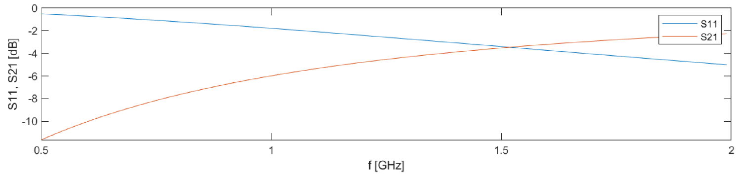
Obr. 3.4: Přenosová charakteristika HP - výstup z aplikace
