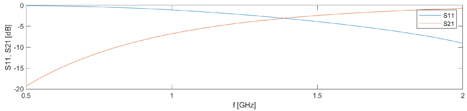
Obr. 3.5: Přenosová charakteristika HP - simulace
