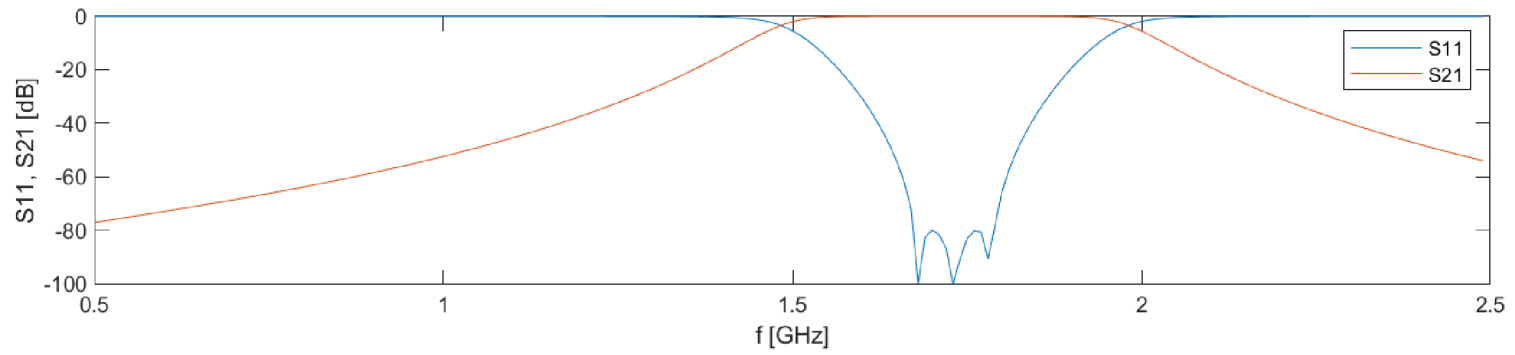
Obr. 3.7: Přenosová charakteristika PP - výstup z aplikace
