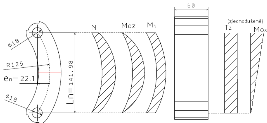
Obrázek 7.15: VVU nůžek
