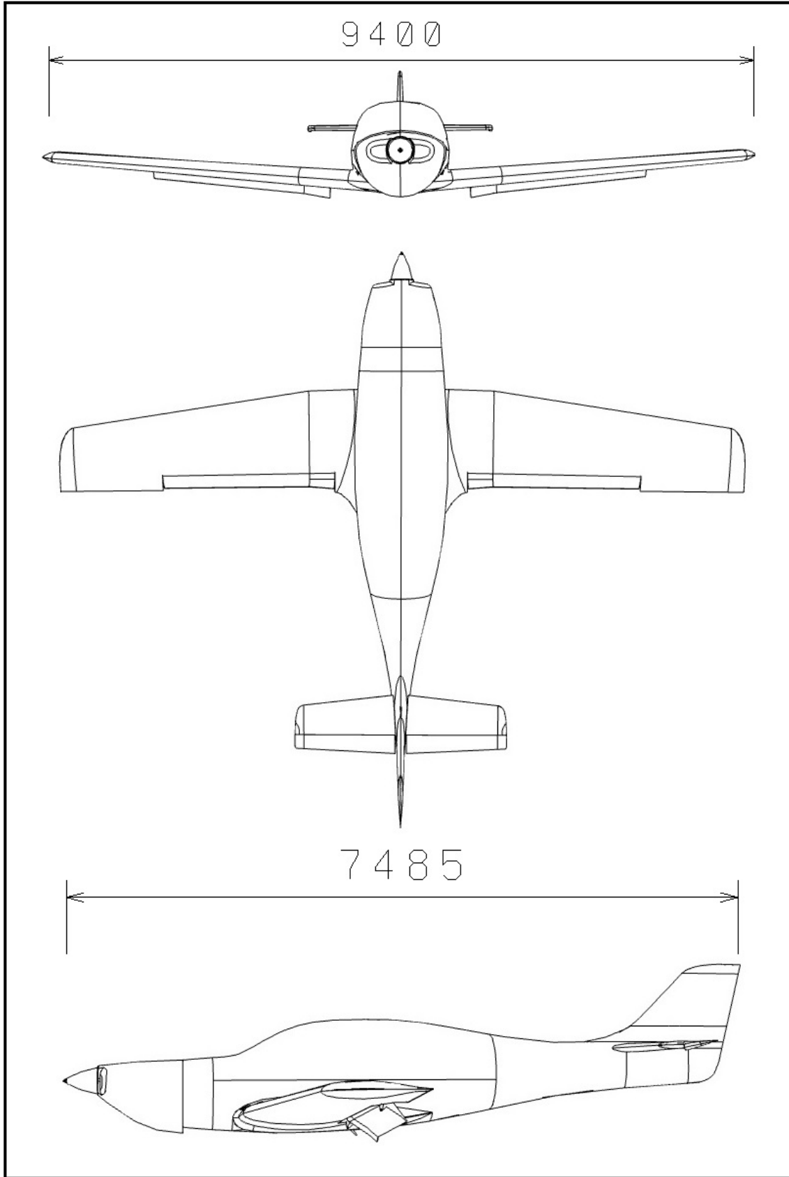
Obrázek 1.3: Muška WT10 Advantic
