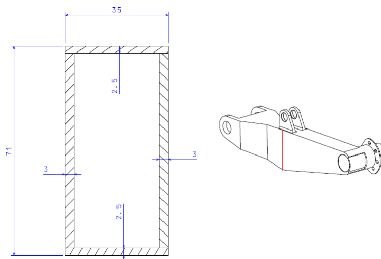
Obrázek 7.3: Průřez vidlice v místě největšího ohybového momentu
