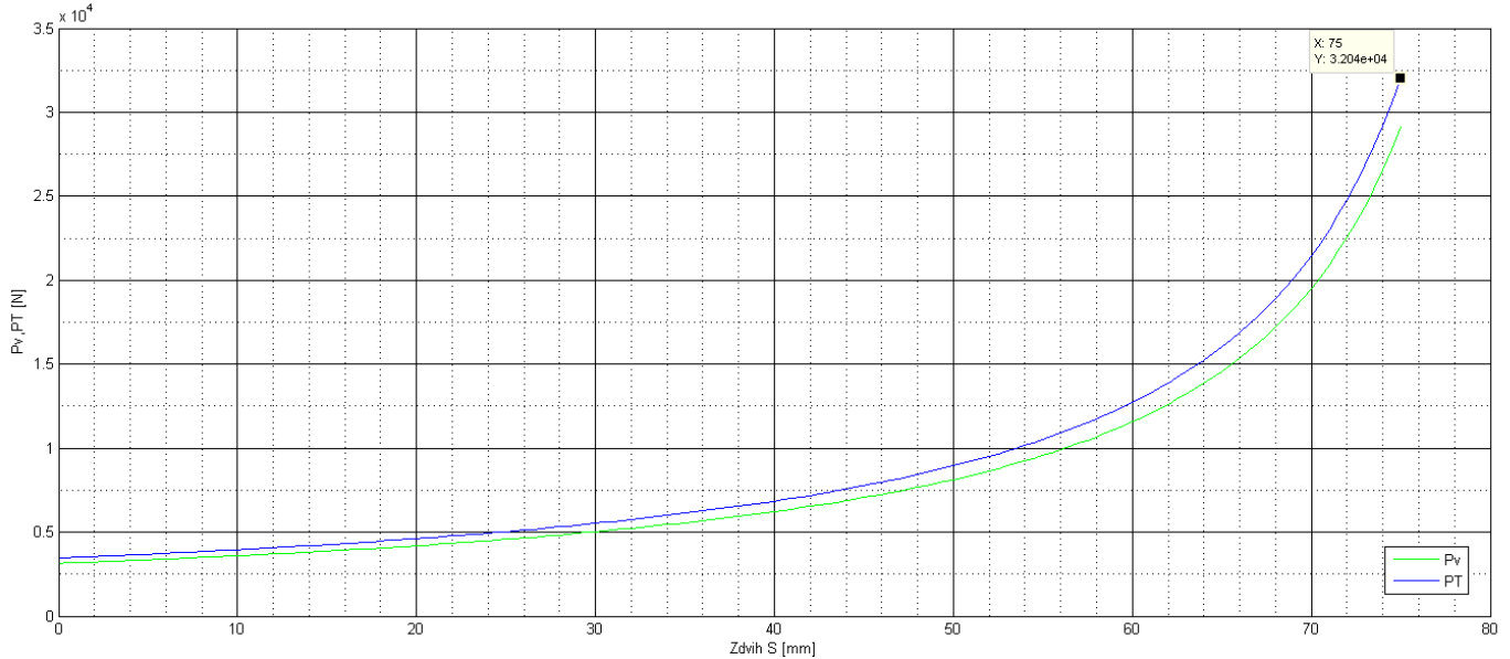
Obrázek 6.5: Křivka tlakové síly polytropického děje a sil vzniklých třením
