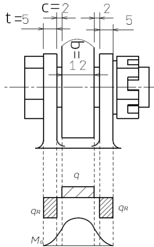
Obrázek 7.5: VVU šroubu spoje vidlice-tlumič: spojitě zatížení q a ohybový moment M_o
