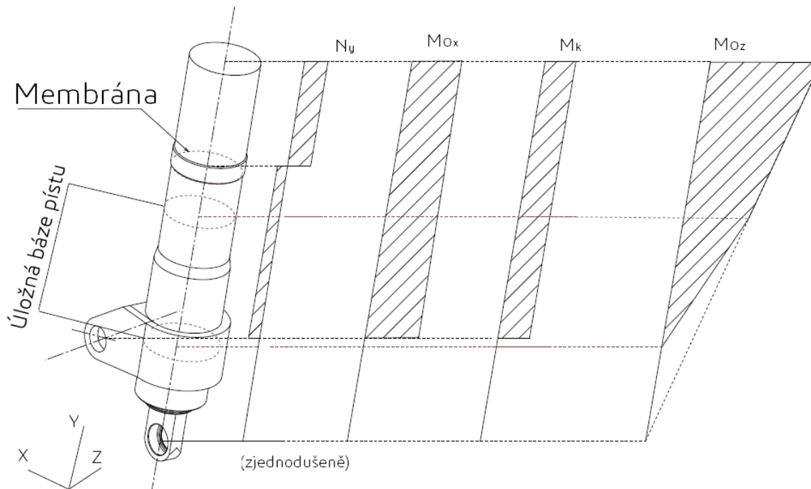
Obrázek 7.8: VUV válce tlumiče při maximálním stlačení pístu tlumiče
