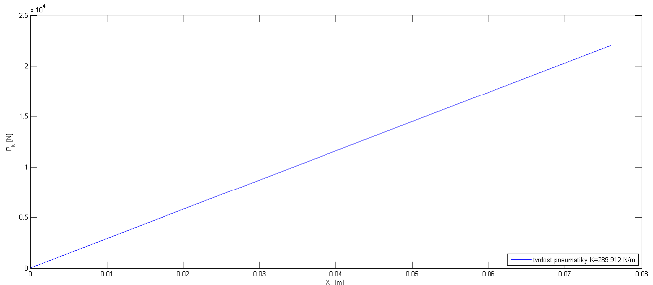
Obrázek 6.8: Přibližný pracovní diagram pneumatiky
