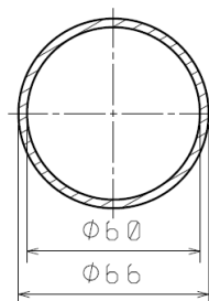
Obrázek 7.19: Průřez nosníku podvozku
