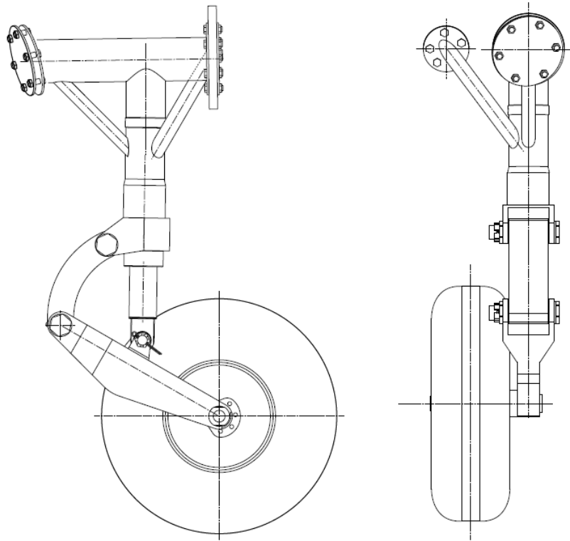
Obrázek 2.1: Nový hlavní podvozek
