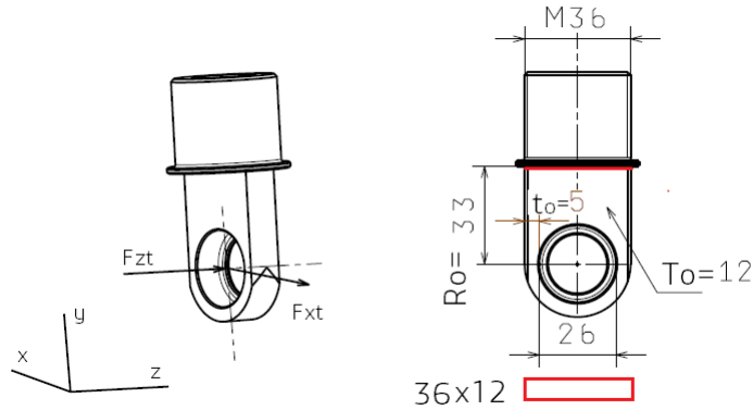
Obrázek 7.13: Pístní oko tlumiče bez ložiska a podložky
