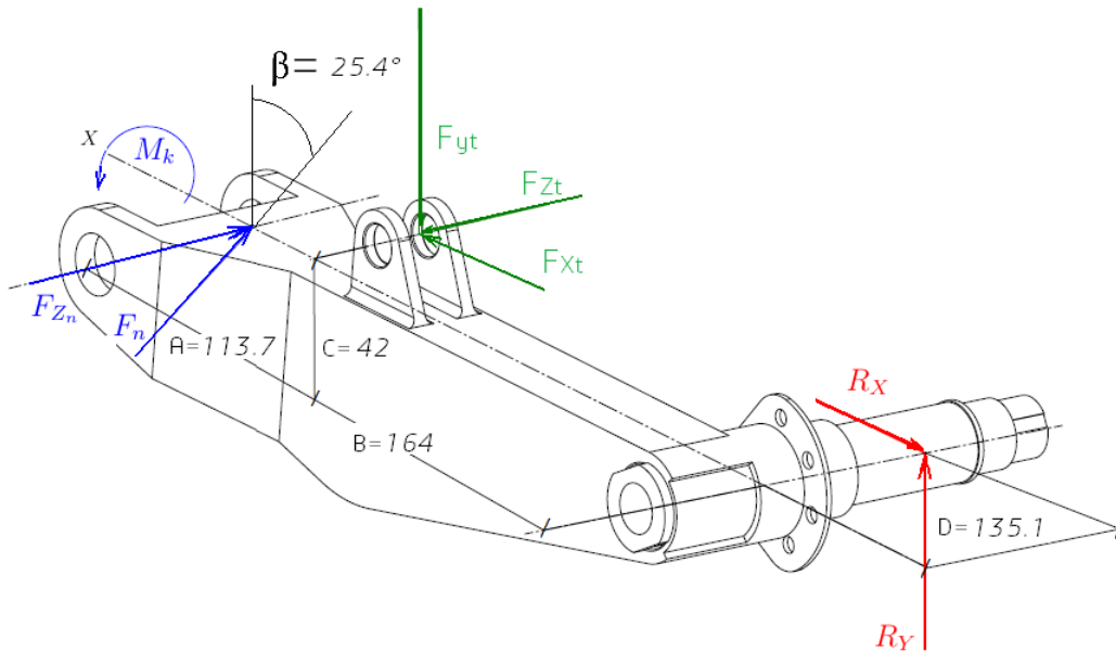
Obrázek 7.1: Působíště jednotlivých sil a momentů na vidlici při maximální stlačení tlumiče
