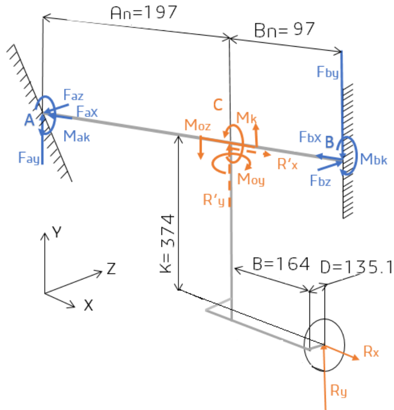
Obrázek 7.17: Schéma nosníku a ostatních části podvozku při stlačeném tlumiči
