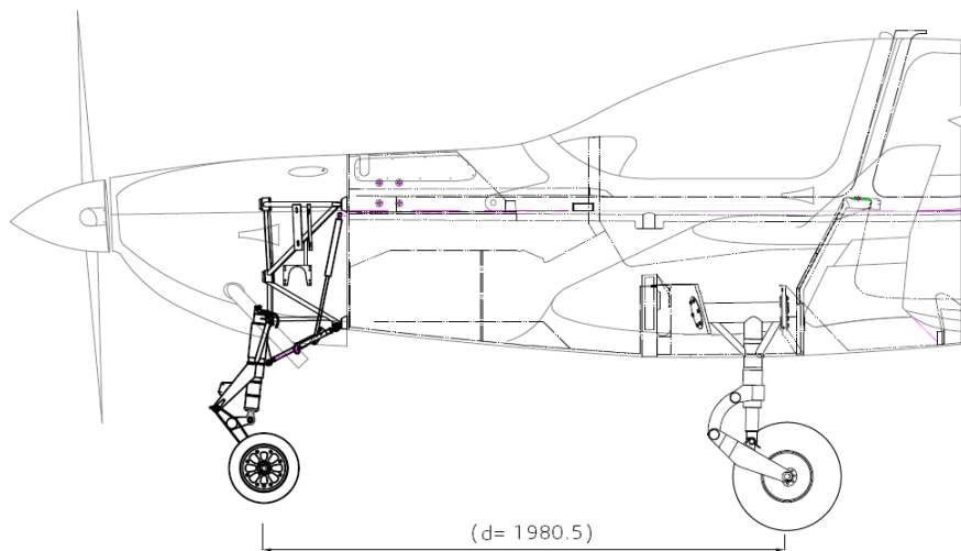
Obrázek 3.2: Nový hlavní podvozek WT10
