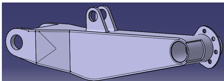
Obrázek 4.4: Vidlice podvozku
