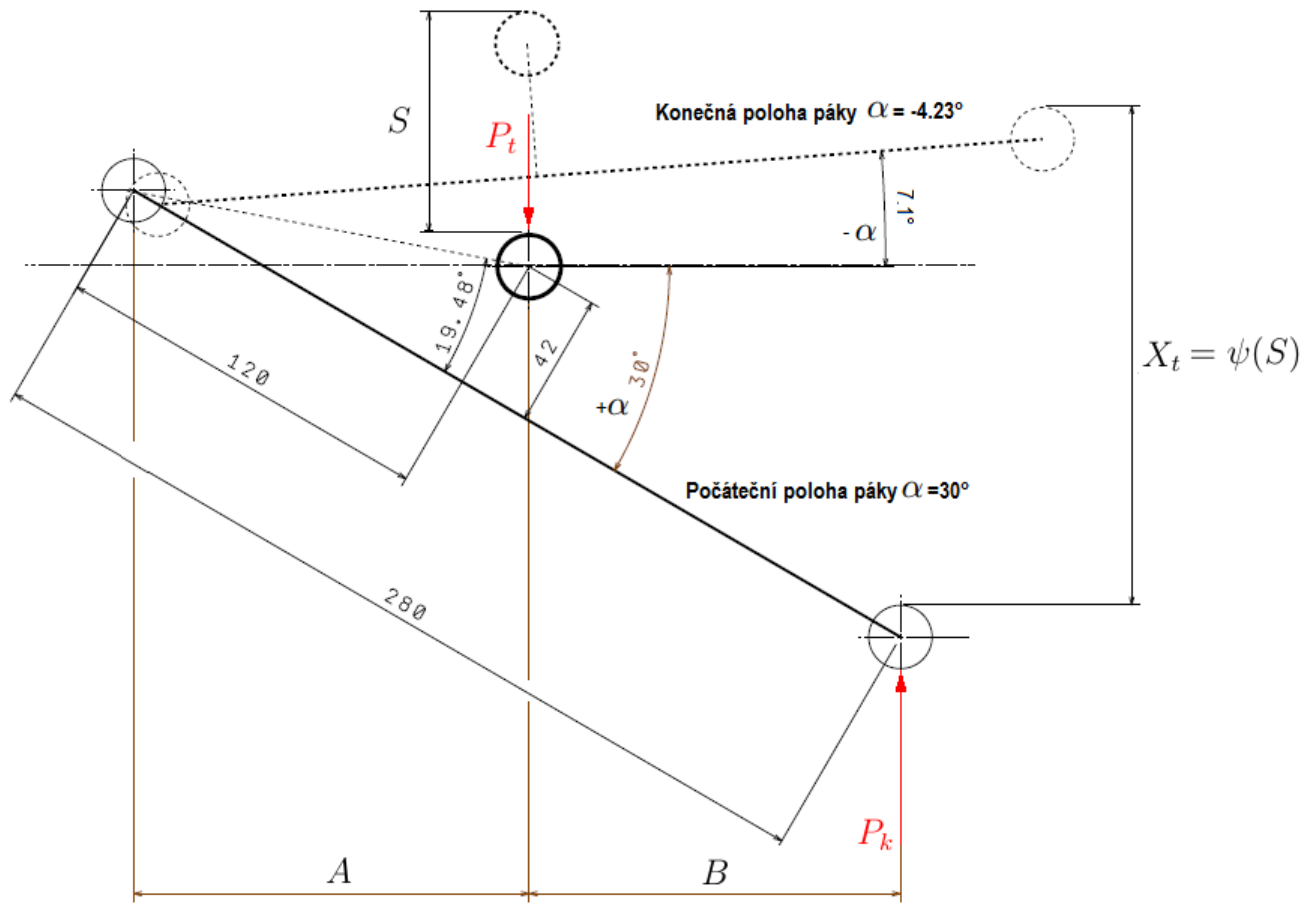
Obrázek 6.3: Kinematika páky hlavního podvozku
