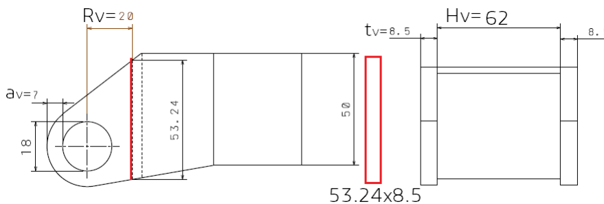
Obrázek 7.14: Oko vidlice připevněné k válci tlumiče
