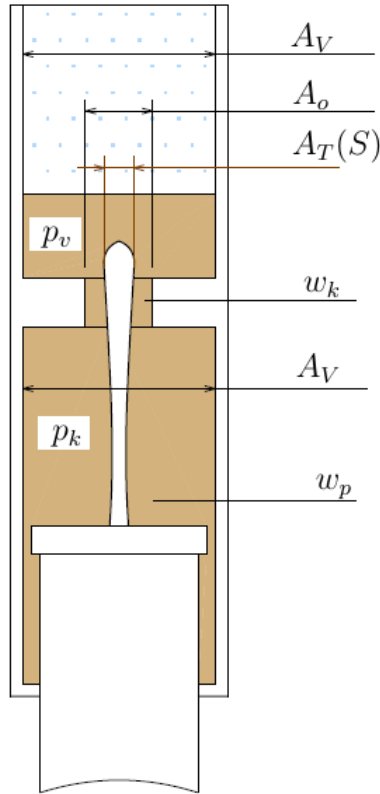
Obrázek 6.12: Jednotlivé stavové veličiny, rychlosti a plochy tlumiče
