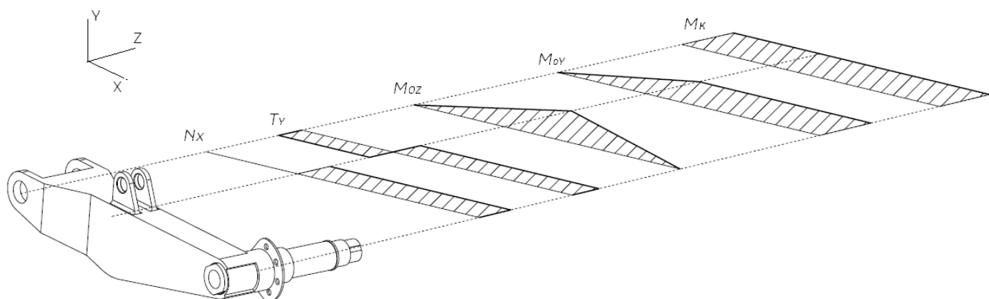
Obrázek 7.2: VUV vidlice
