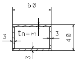
Obrázek 7.16: Kritický průřez nůžek
