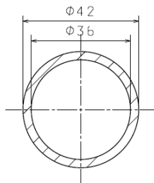
Obrázek 7.12: Průřez pístní tyče tlumiče v místě největšího zatížení
