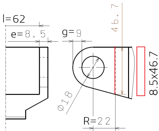
Obrázek 7.6: Rozměry oka vidlice spoje vidlice-nůžky
