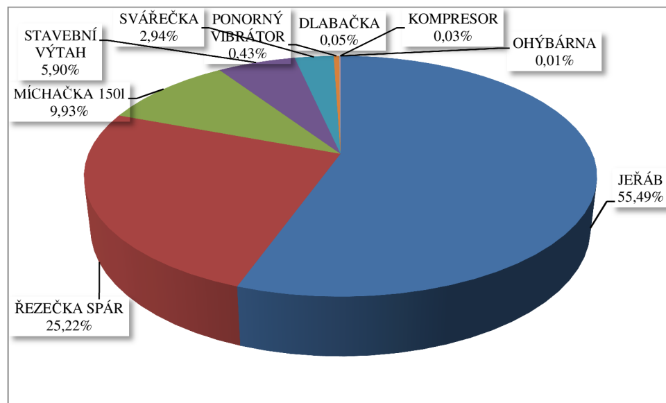
Obrázek 19 – Graf celkové spotřeby strojů
