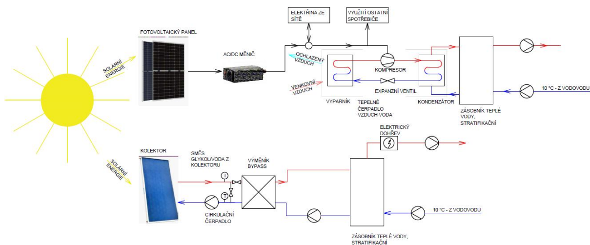
Obrázek 17: Schéma simulace
