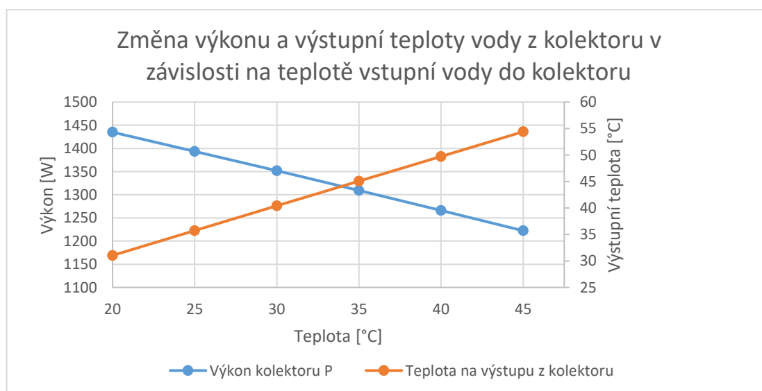
Obrázek 23: Závislost parametrů kolektoru na vstupní teplotě vody
