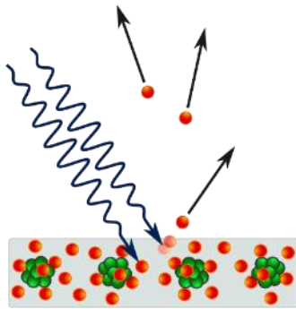
Obrázek 4 Fotoelektrický jev [12]
