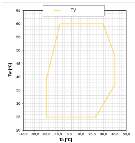
Obrázek 21 Pracovní oblast přípravy TV [54]
