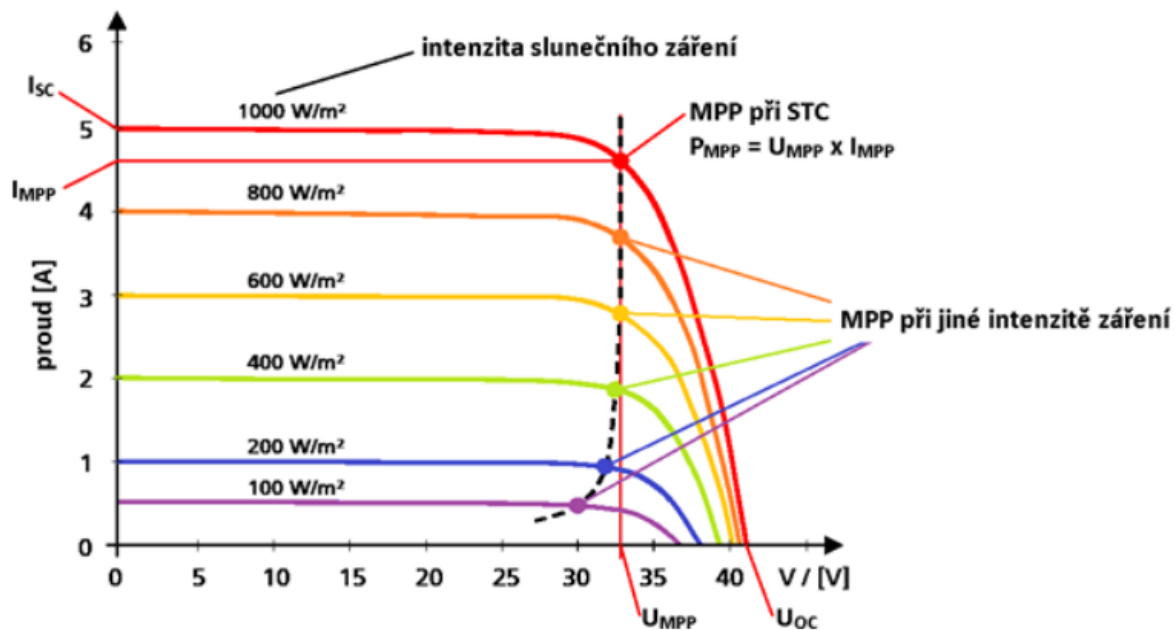
Obrázek 6 Poloha MPP [23]
