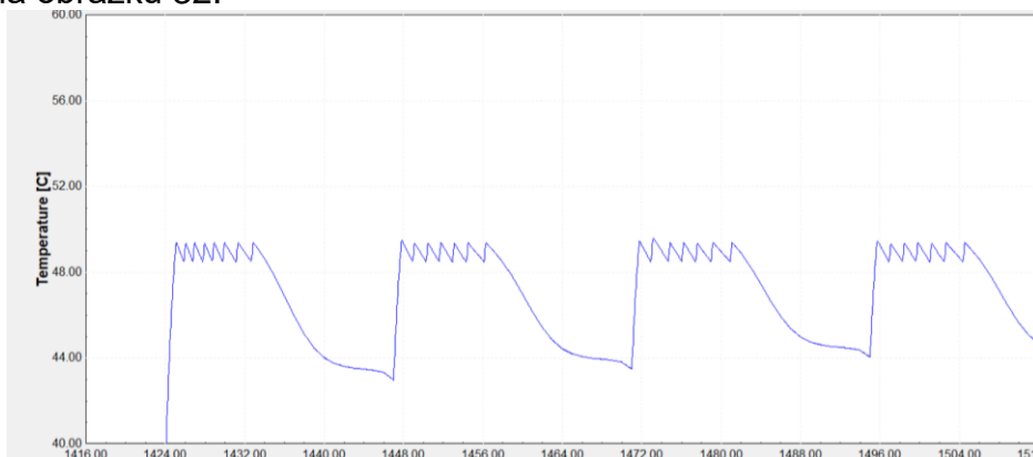
Obrázek 32 Průběh teplot v zásobníku soustavy PVTČ
