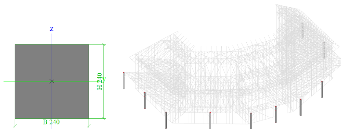
Obrázek 13 Balkonové sloupy 240x240 mm
