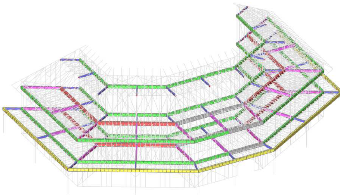
Obrázek 14 Průvlaky
