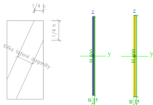
Obrázek 19 Příklad průřezů fiktivních prutů
