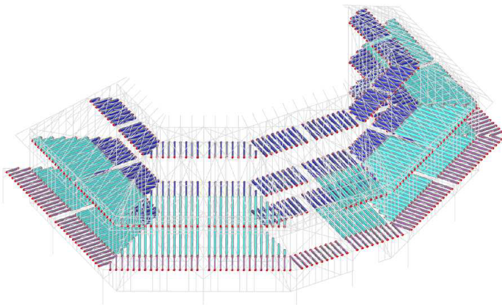
Obrázek 16 Stropnice
