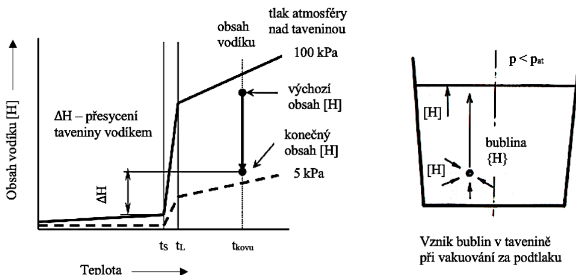
Obrázek 18: Princip vakuového odplyňování [4]
