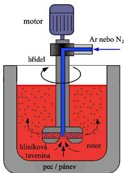
Obrázek 22: Schéma FDU [21]
